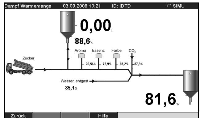
Prozessbild
