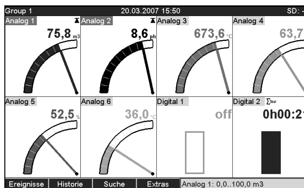
Instrumentendarstellung
