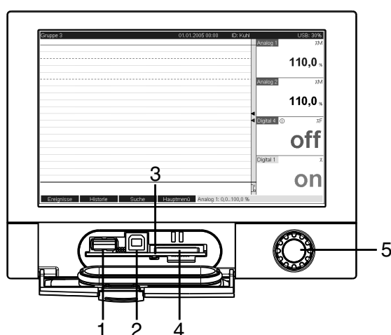
Gerätefront mit geöffneter Klappe/Tastatur
