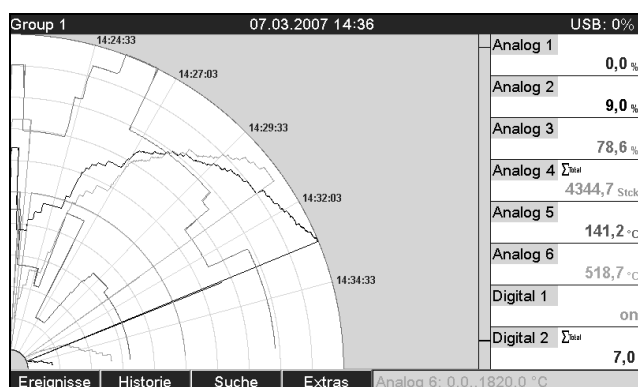
Kreisblattdarstellung
