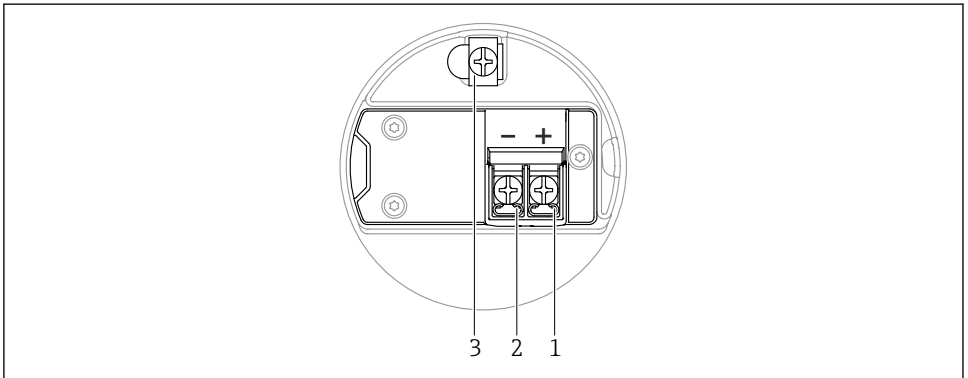
图 4 接线腔中的接线端子和接地端
