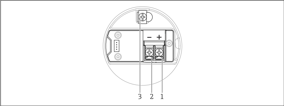
图 5 接线腔中的接线端子和接地端
