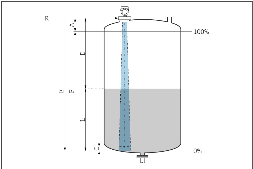
图 11 液位测量的设置参数
