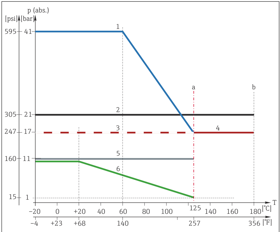
图 14 温压曲线
