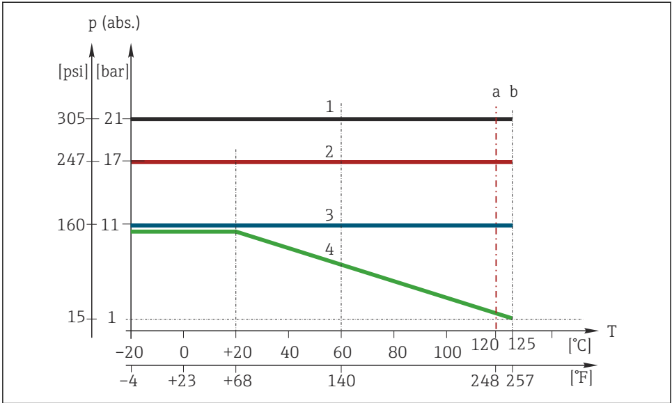
图 12 温压曲线
