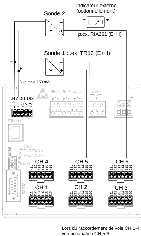
Fig. 6 : Raccordement de la sortie tension auxiliaire utilisée comme alimentation de transmetteur (MUS) pour capteurs 4 fils dans la gamme de courant
