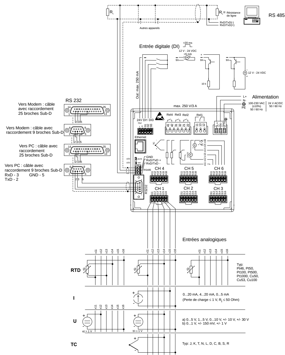
Fig. 4: Schéma électrique
