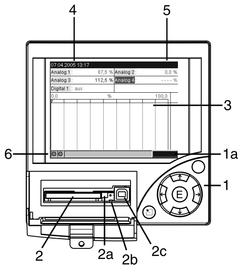
Abb. 7: Geräteanzeige / Bedieneinheiten
