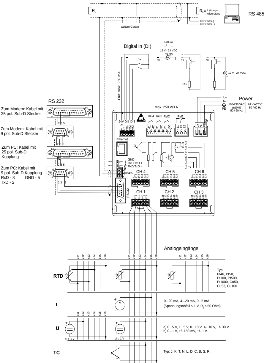
Abb. 4: Schaltplan
