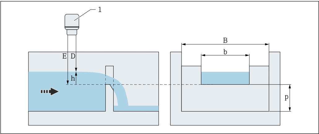
146 Kronenhöhe im Rechteckwehr mit scharfer Krone (ISO 1438)
