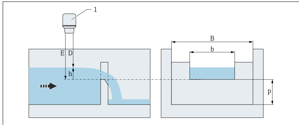
110 Wehrtyp: Rechteckwehr mit scharfer Krone (ISO 1438)
