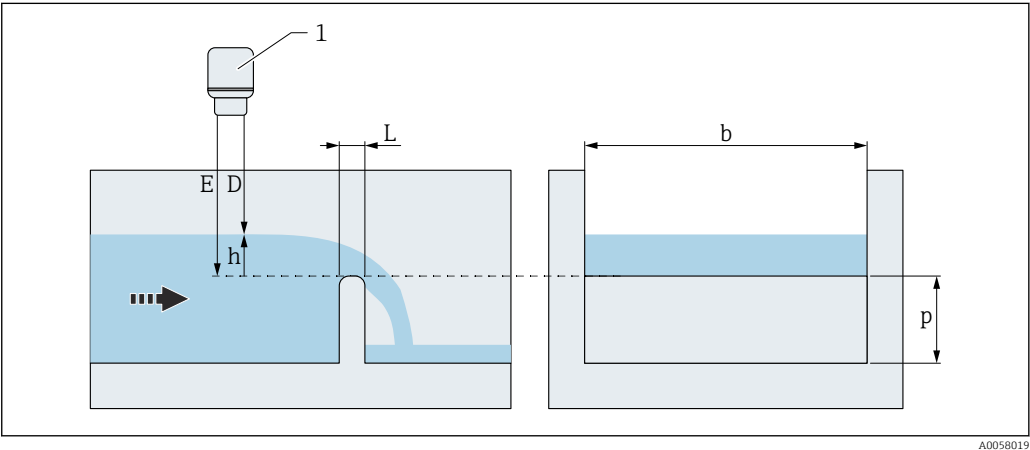
108 Wehrtyp: Horizontales Wehr mit abgerundeter Krone (ISO 4374)
