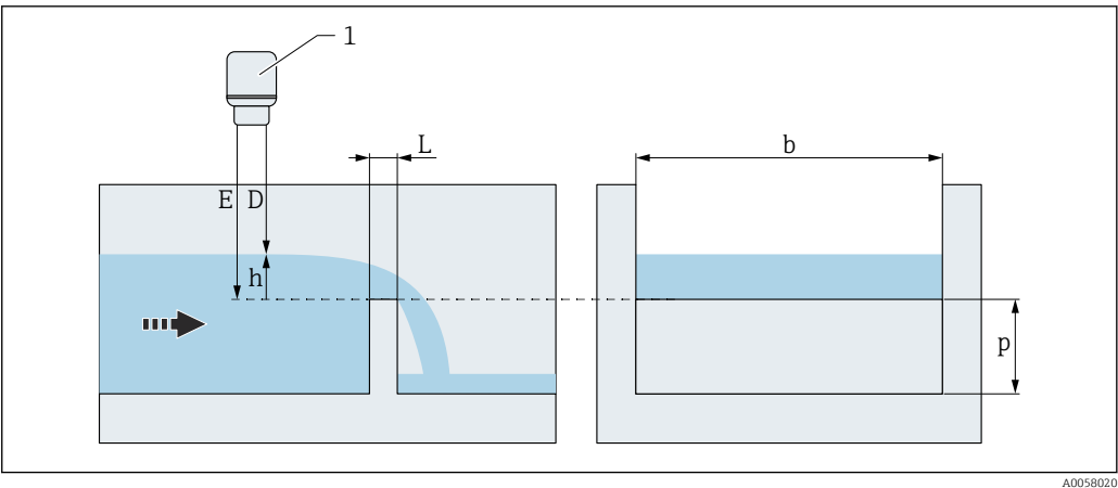
109 Wehrtyp: Rechteckiges breitkroniges Wehr (ISO 3846)
