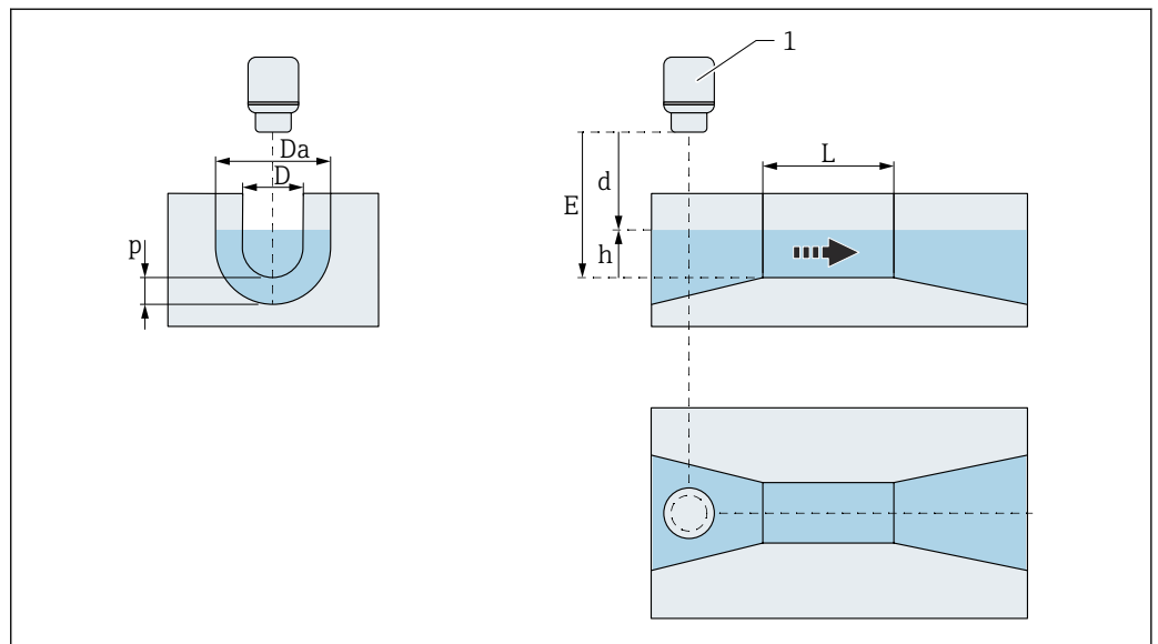
119 Zulaufdurchmesser Da in der U-Form-Rinne (ISO 4359)
