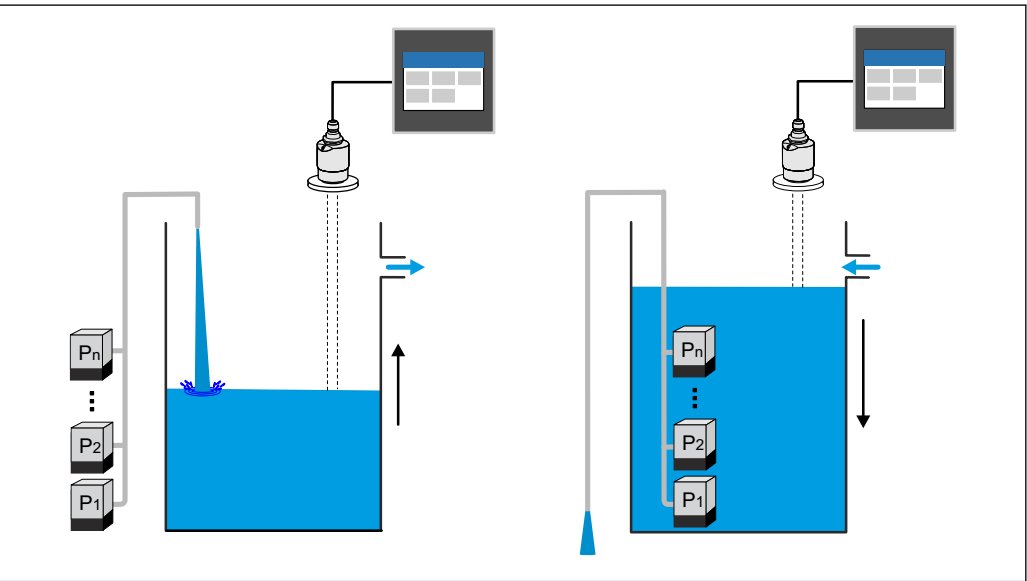
3 Betriebsart Pumpensteuerung
