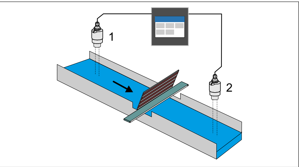
4 Betriebsart Rechensteuerung
