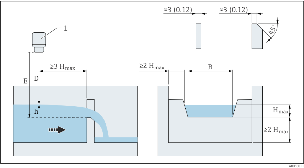
107 Wehrtyp: Trapezwehr
