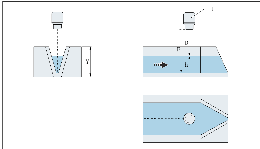
106 Gerinnetyt: H-Rinne
