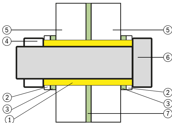
Verwendung des Stutzenisolationssets
