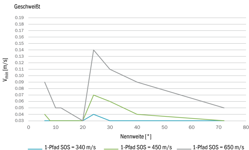
Bild 67 V_{\min} bei 20 % Unsicherheit von 1-Pfad-Lösungen abhängig von der Schallgeschwindigkeit (SOS)
