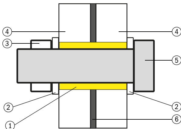
Verwendung der Zentrierhülsen
