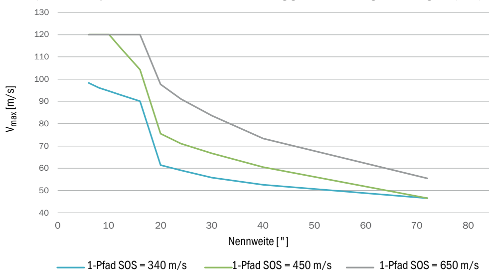
Bild 66 Exemplarische V_{\max} von 1-Pfad-Durchstrahlern, abhängig von der Schallgeschwindigkeit (SOS)
