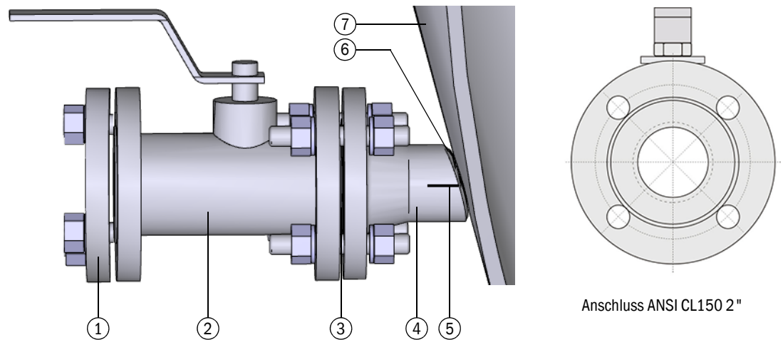
Bild 16 Montagezubehör (am Beispiel ANSI CL150)
