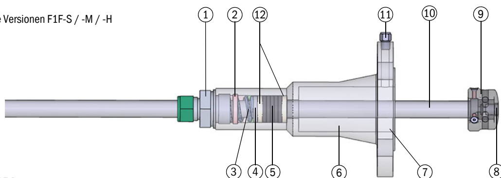
Bild 8 Prozessgasberührte Teile
