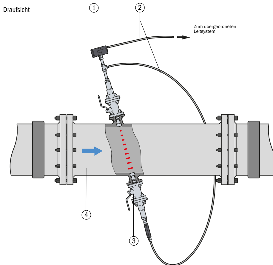
Systemübersicht FLOWSIC100 Flare-XT Transmitter
