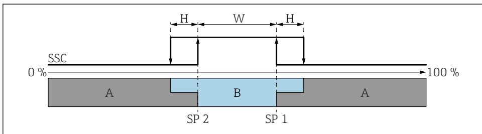
图 10 SSC，双区间控制
