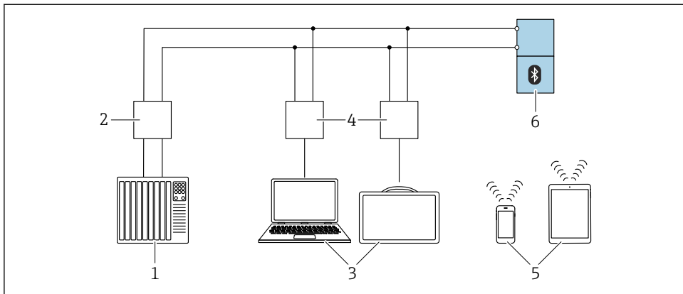
图 5 通过 IO-Link 进行远程操作
