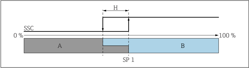
图 9 SSC, 单点
