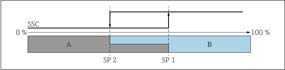
图 8 SSC, 两点
