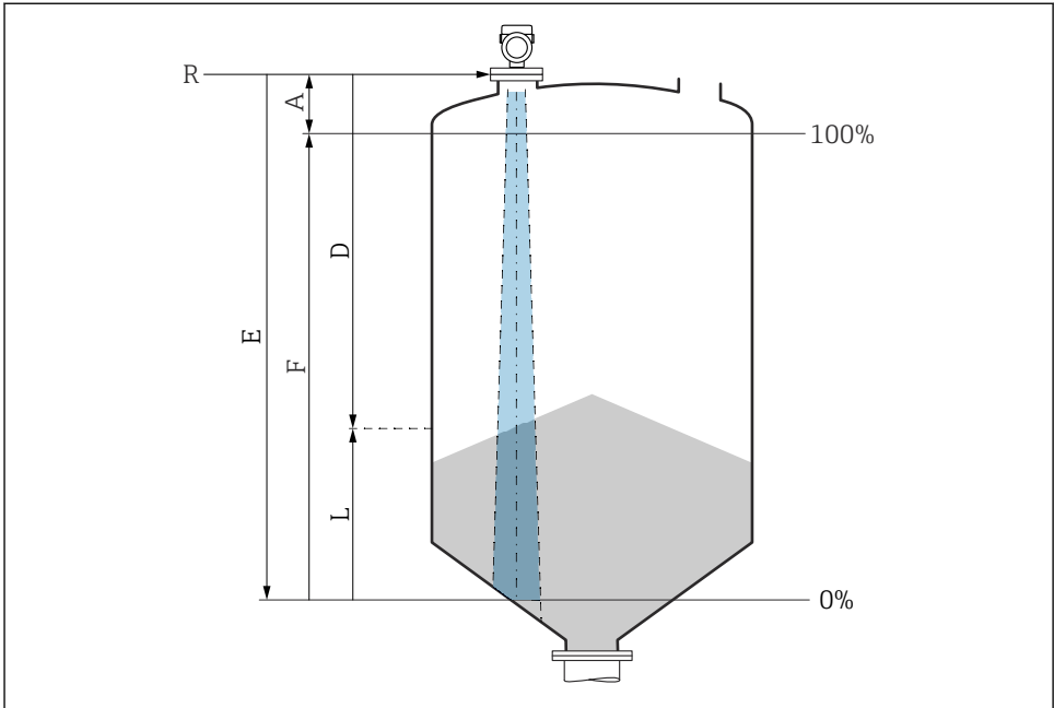
图 7 固体散料料位测量的设置参数
