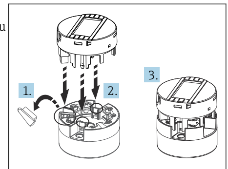
13 Enfiler l'afficheur sur le transmetteur
