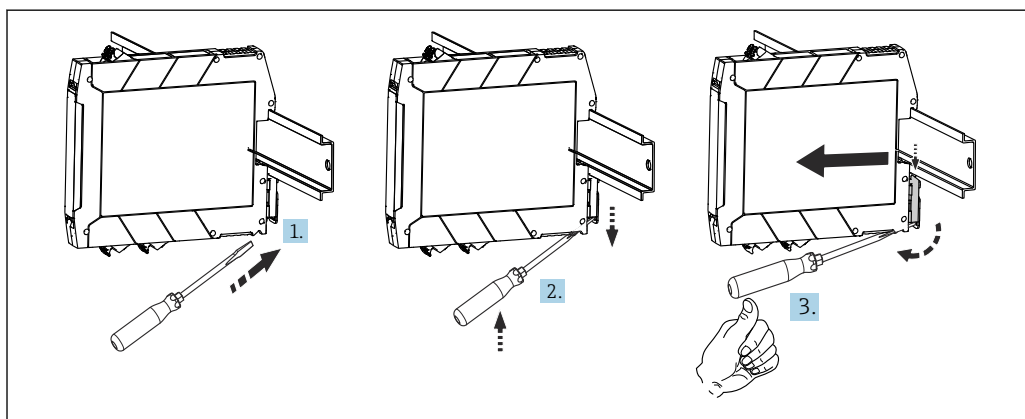
5 Démontage du transmetteur pour rail DIN
