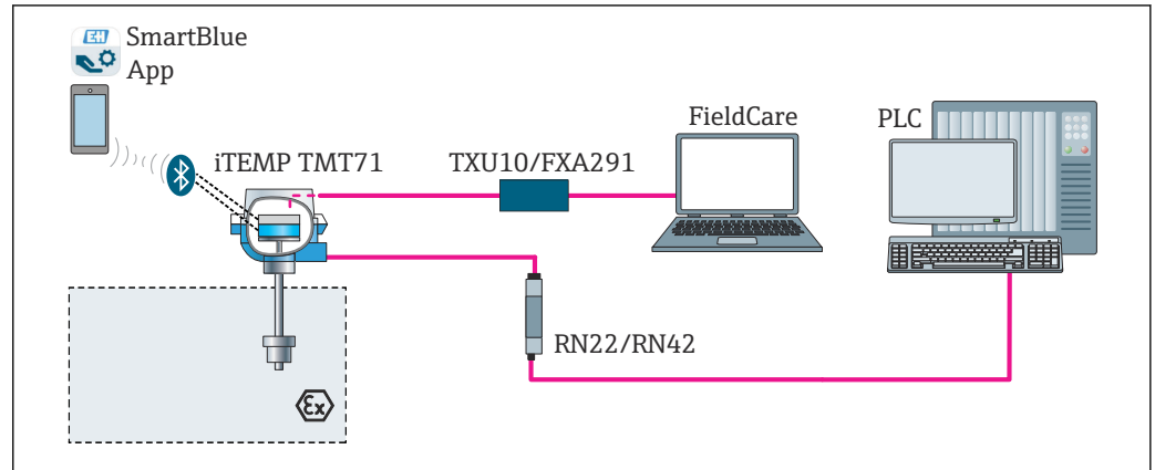
12 Options de configuration pour le transmetteur via l'interface CDI
