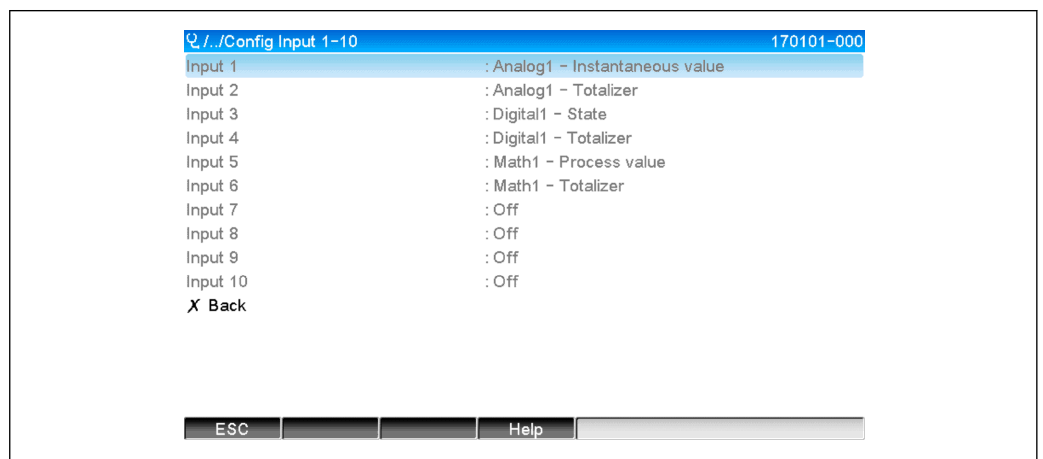
24 Visualisering av undermenyn Konfig ingång 1-10 (lokal drift)
