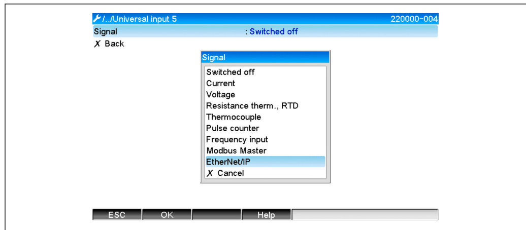
16 EtherNet/IP som insignal
