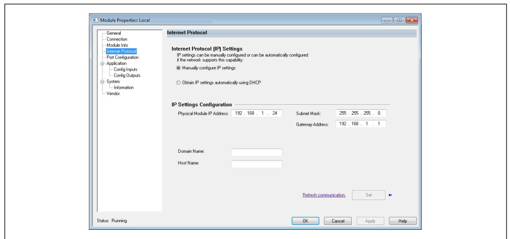
38 Internetprotokollsida: Konfigurera IP-inställningar
