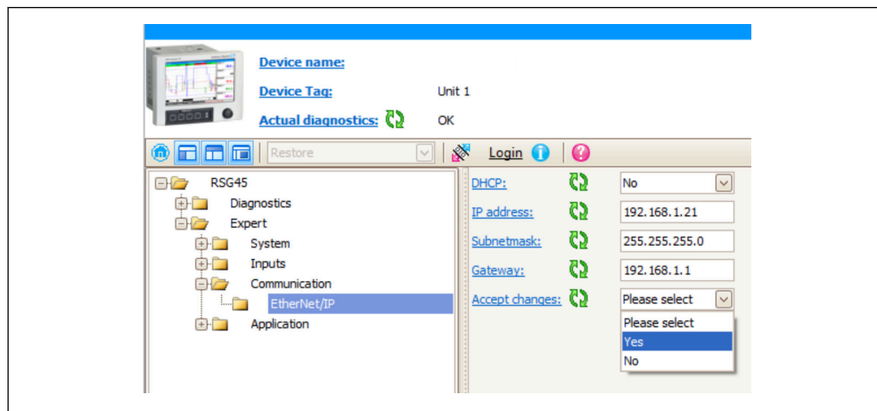
12 Nätverksinställningar: acceptera ändringar (DTM)
