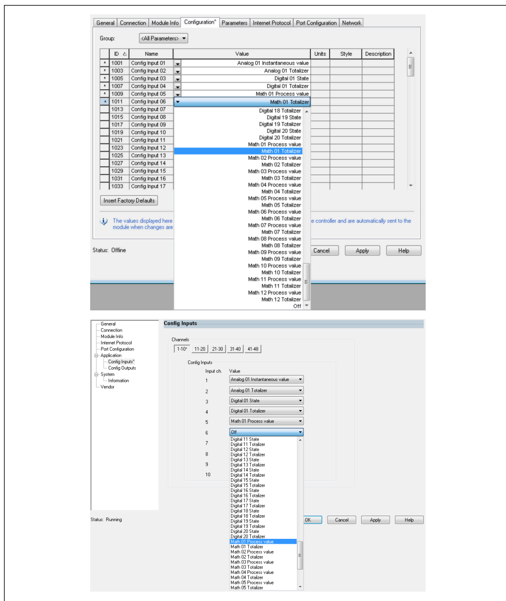
18 Konfigurering av ingångs-/utgångsdata med hjälp av konfigurationsenhet (EDS AOP/Kundanpassad AOP)
