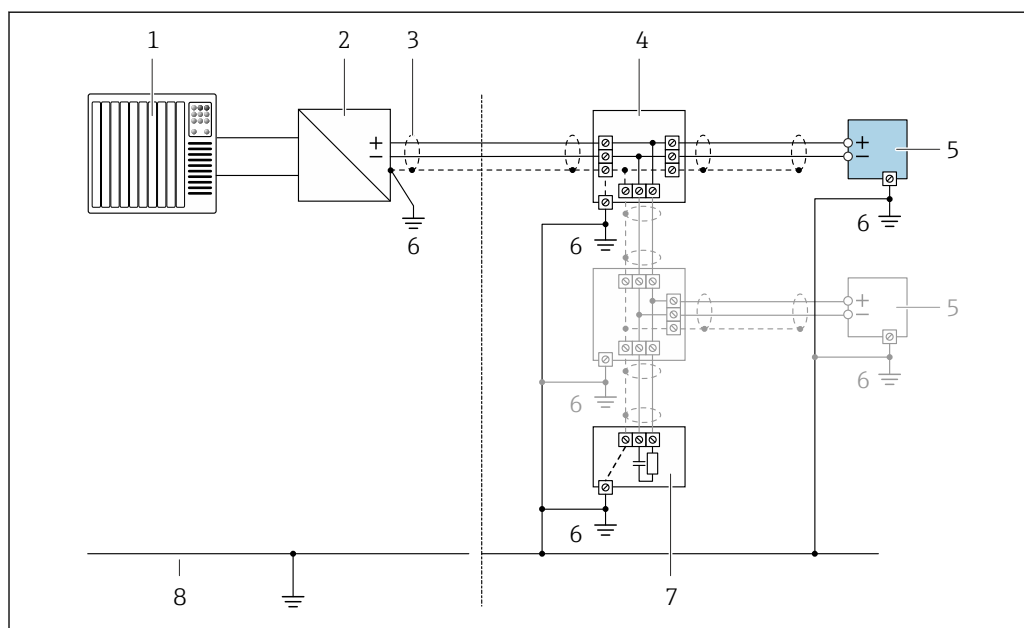
11 FOUNDATION フィールドバスの接続例
