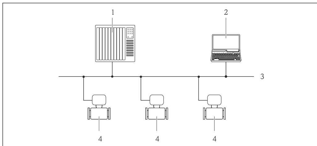
図 60 PROFIBUS DP ネットワークを介したリモート操作のオプション
