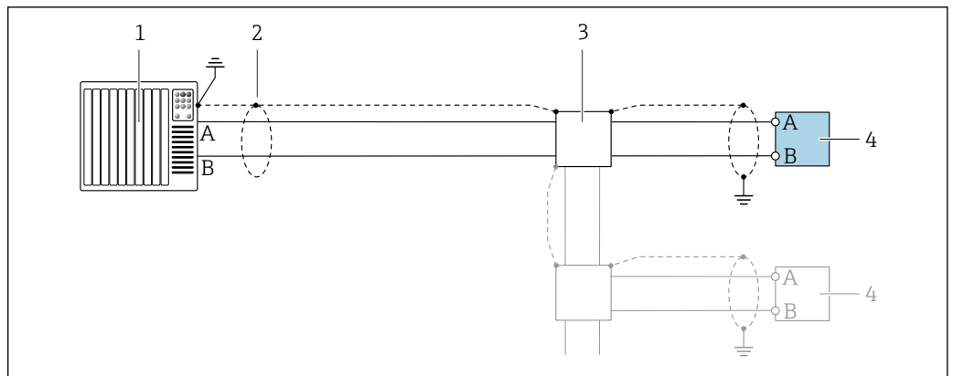
図 12 Modbus RS485（非危険場所および Zone 2/Div. 2 用）の接続例
