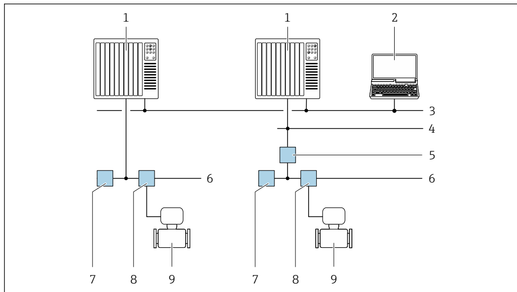
図 59 FOUNDATION フィールドバスネットワークを介したリモート操作のオプション
