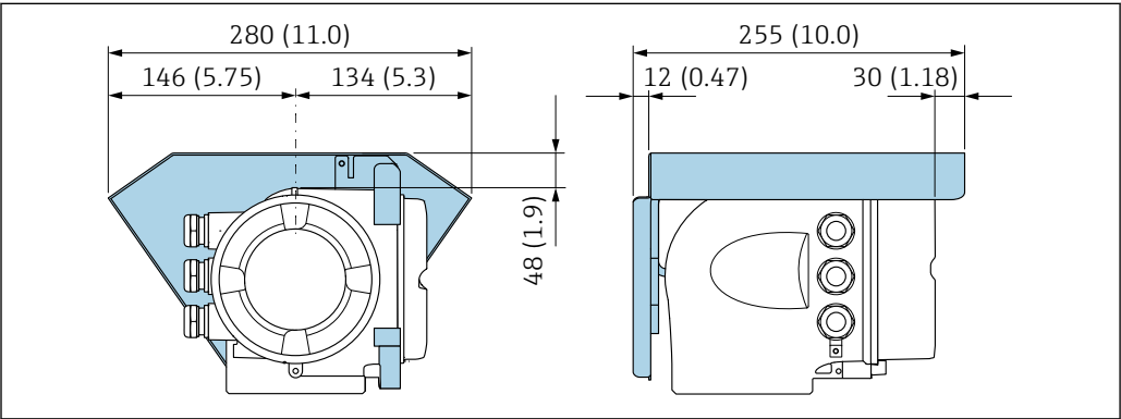
図 50 Proline 500 用の日除けカバー、単位 mm (in)
