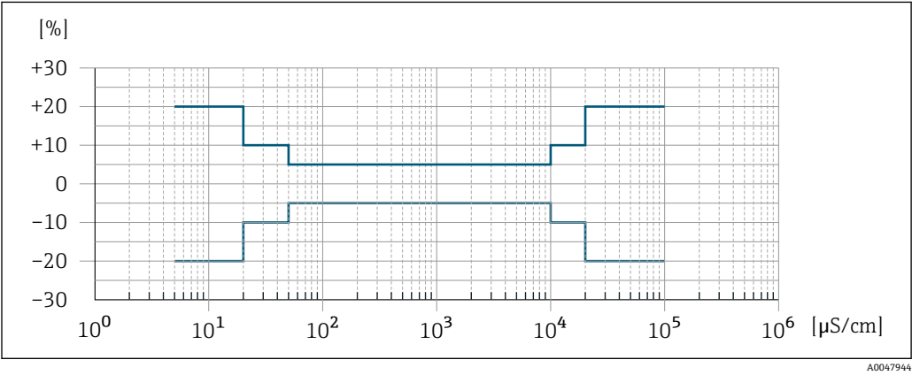
図 26 測定誤差（オプション：「校正された導電率測定」のオーダーコード、オプション CW）
