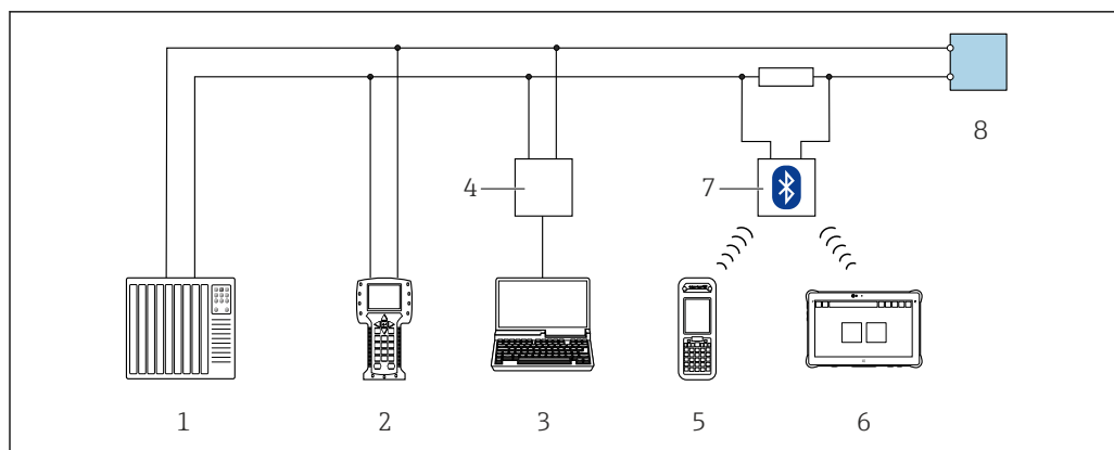
図 57 HART プロトコル経由のリモート操作オプション (アクティブ)
