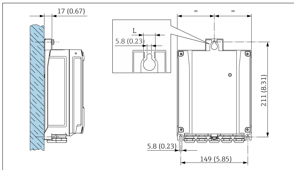
図 29 単位 mm (in)
