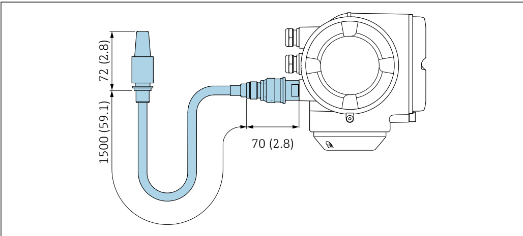
図 54 単位 mm (in)
