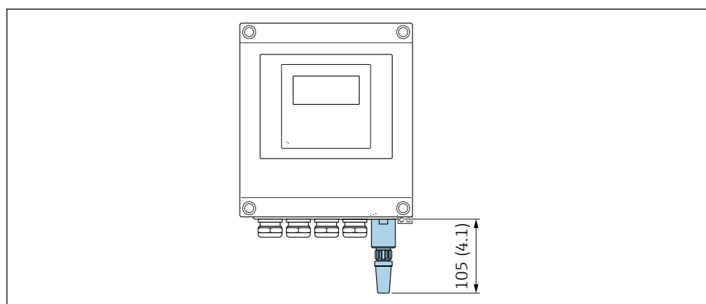
図 45 単位 mm (in)
