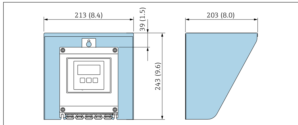
図 32 Proline 500 – デジタル用の日除けカバー、単位 mm (in)
