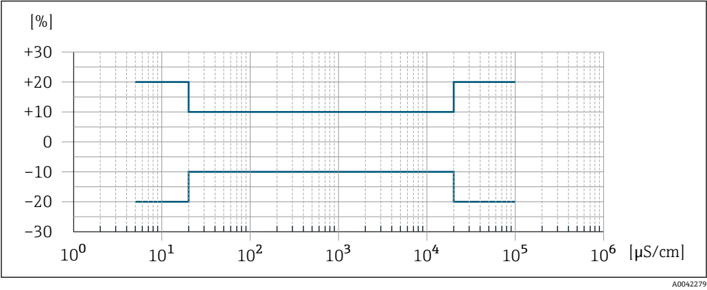
図 25 測定誤差（標準）
