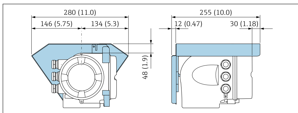
図 44 Proline 500 用の日除けカバー、単位 mm (in)
