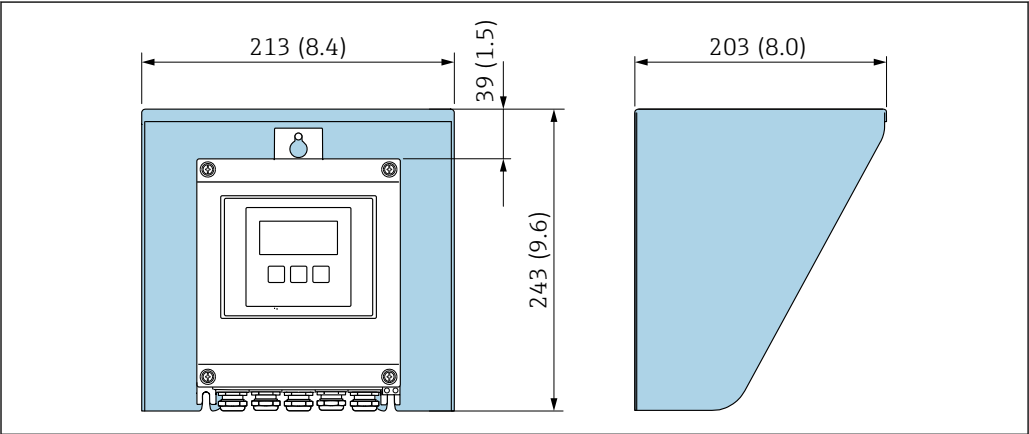
図 49 Proline 500 – デジタル用の日除けカバー、単位 mm (in)
