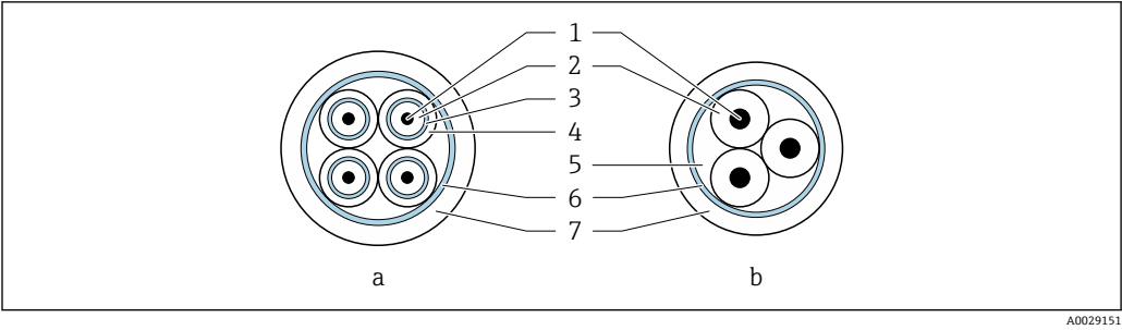
図 22 ケーブル断面
