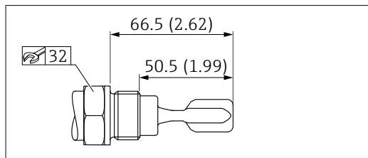
図 23 ISO 228 G ¾ ネジ接続。測定単位 mm (in)
