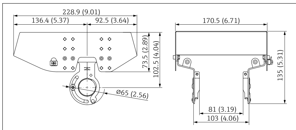
40 日除けカバー、SUS 316L 相当、XW112 の寸法。測定単位 mm (in)
