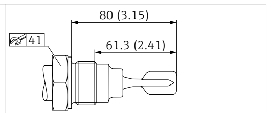
図 24 ISO 228 G 1 ネジ接続。測定単位 mm (in)
