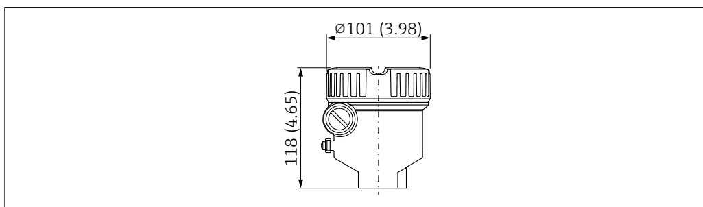
16 シングルコンパートメントハウジング、アルミニウム、コーティングの寸法 (Ex d/XP、粉塵防爆に適合、ハウジングカバーに窓なし)。測定単位 mm (in)
