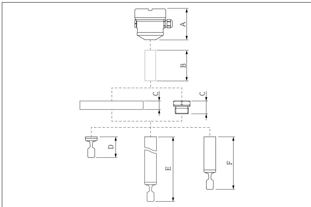
図 13 本体高さを計算するための構成品
