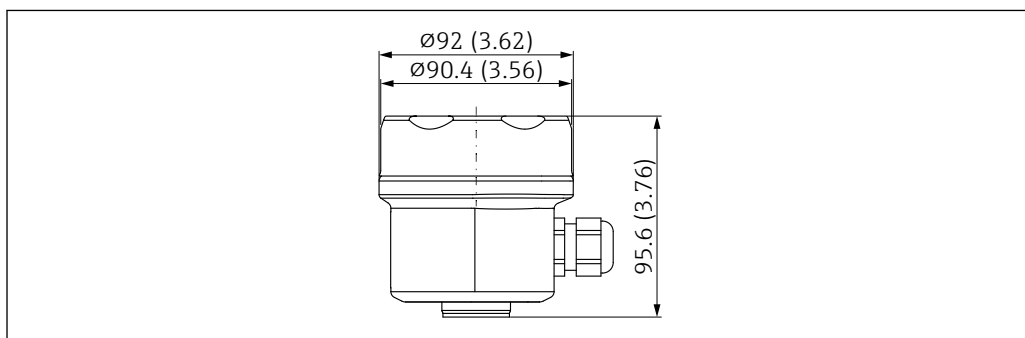
17 シングルコンパートメントハウジング、SUS 316L 相当、サニタリ仕様の寸法（ハウジングカバーに窓なし）。測定単位 mm (in)
