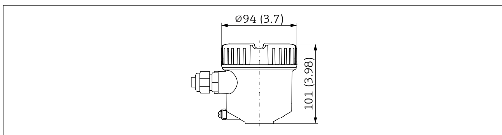
図 14 シングルコンパートメントハウジング、プラスチックの寸法 (ハウジングカバーに窓なし)。測定単位 mm (in)
