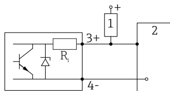
9 Tilkoblingseksempel for den digitale inngangen
