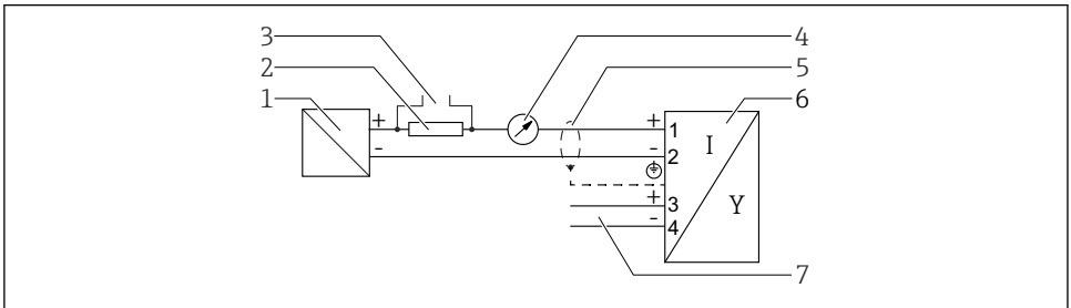
7 Funksjonsdiagram 4 – 20 mA HART, bryterutgang
