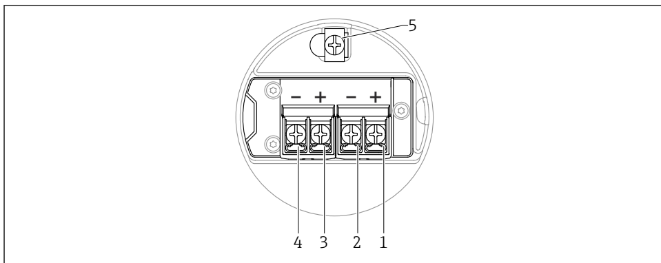
14 Klemmetilordning i tilkoblingsrom; 4 – 20 mA HART, bryterutfgang, hus med dobbeltrom
