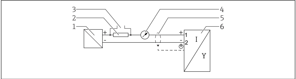
6 Funksjonsdiagram 4 – 20 mA HART
