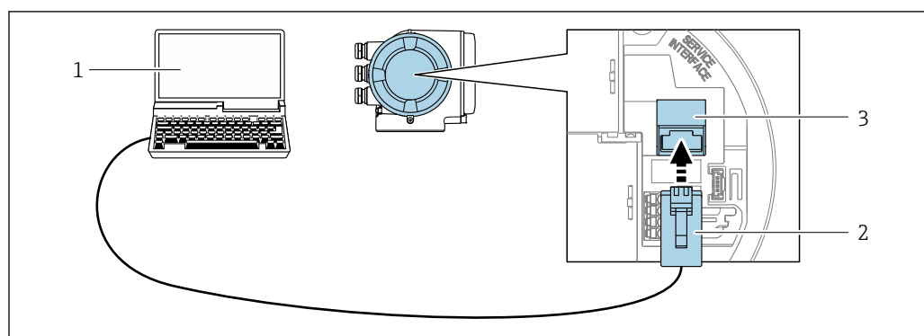
54 Conexão através de Interface de operação (CDI-RJ45)
