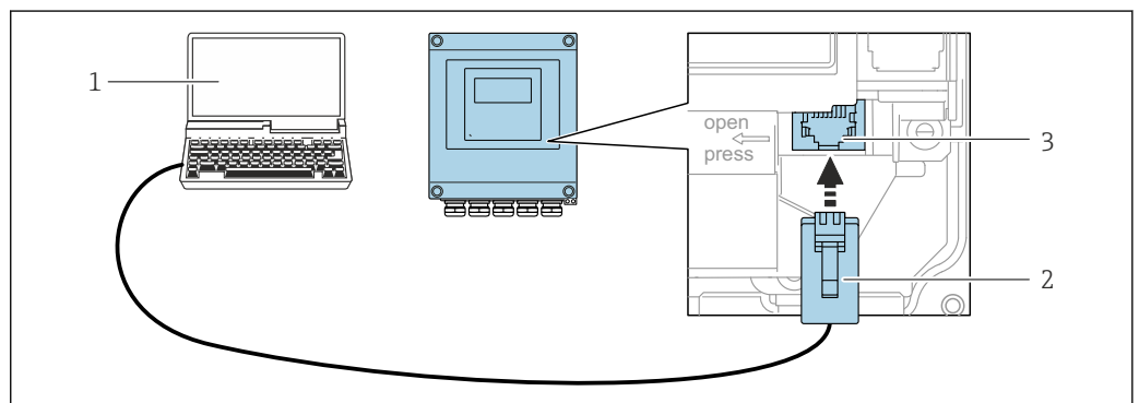
53 Conexão através de Interface de operação (CDI-RJ45)
