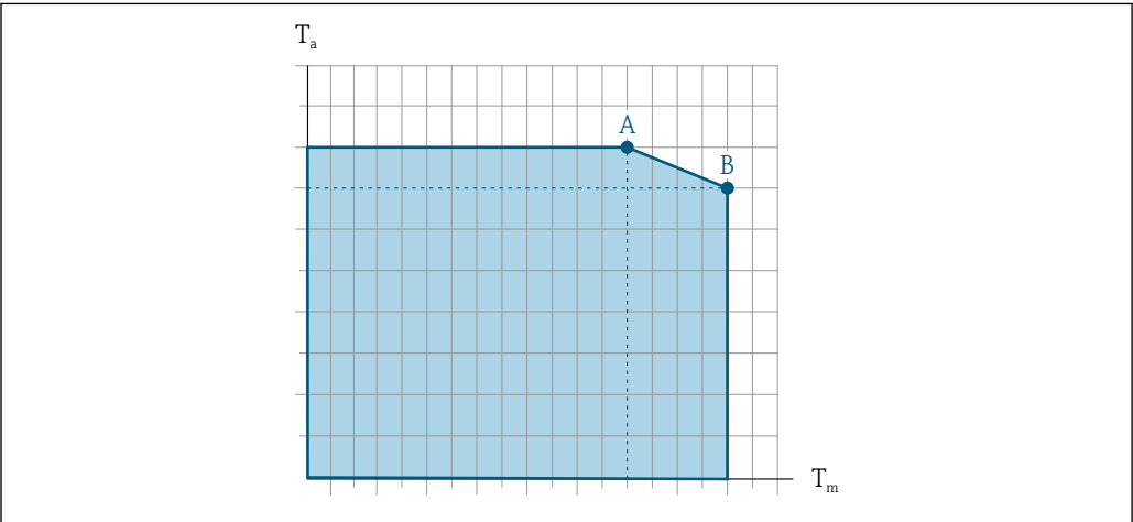
21 Representação exemplar, valores na tabela abaixo. T_a Temperatura ambiente T_m Temperatura do meio A Temperatura máxima permitida do meio T_m a T_{a\text{máx.}} = 60\text{ °C (140 °F)} ; temperaturas do meio mais altas T_m requerem uma redução na temperatura ambiente T_a B Temperatura ambiente T_a máxima permitida para a temperatura média T_m máxima especificada do sensor
