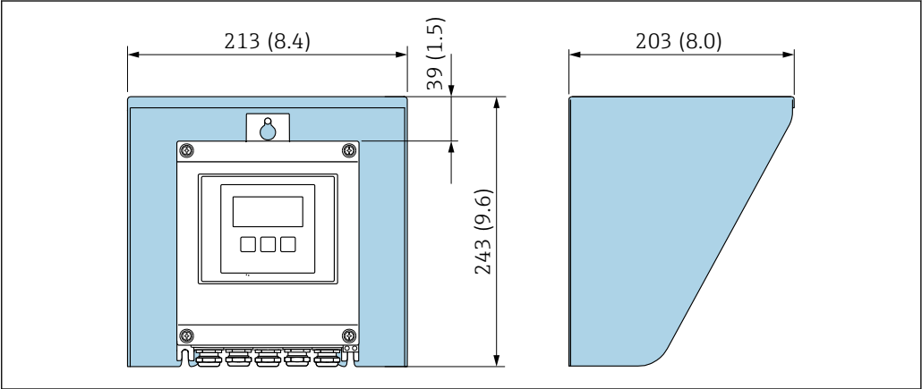
33 Tampa de proteção contra tempo para Proline 500 - digital; unidade mm (pol.)
