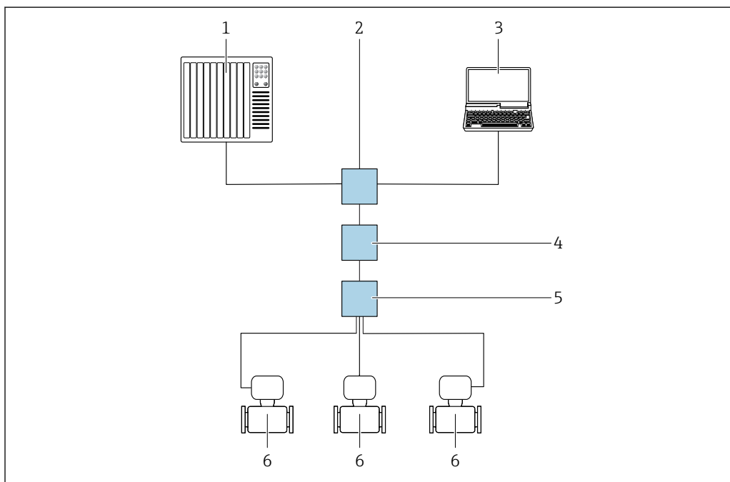
51 Opções para operação remota através do protocolo Modbus TCP por Ethernet-APL (ativa)
