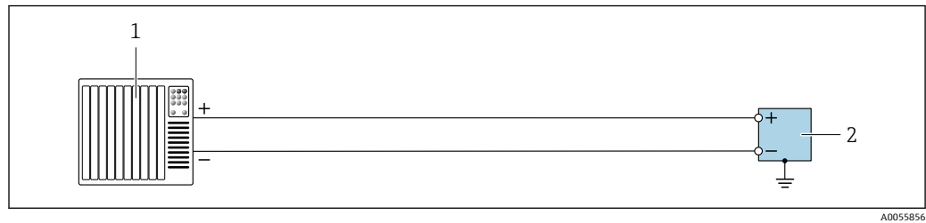
図 21 パルス出力/周波数出力/スイッチ出力（アクティブ）の接続例
