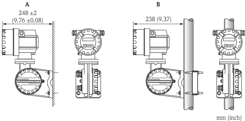
Fig. 1: Montagem do transmissor (versão remota)
