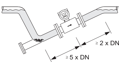
Instalação em uma tubulação parcialmente preenchida
