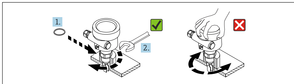
15 Uvrtanje uređaja
