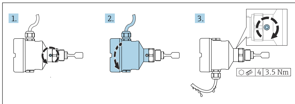
17 Kućište s vanjskim vijkom za blokiranje i petljom za kapanje
