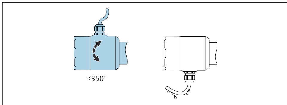
16 Kućište bez vijka za zaključavanje s omčom za kapanje
