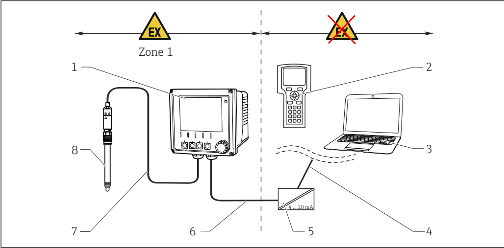
図 55 危険場所 JPN での設置
