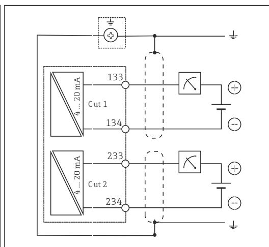
図 13 配線図
