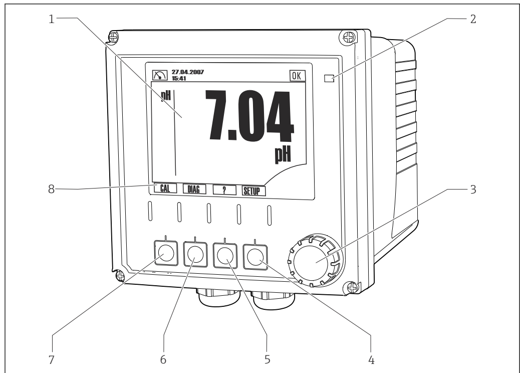
図 63 操作の概要
