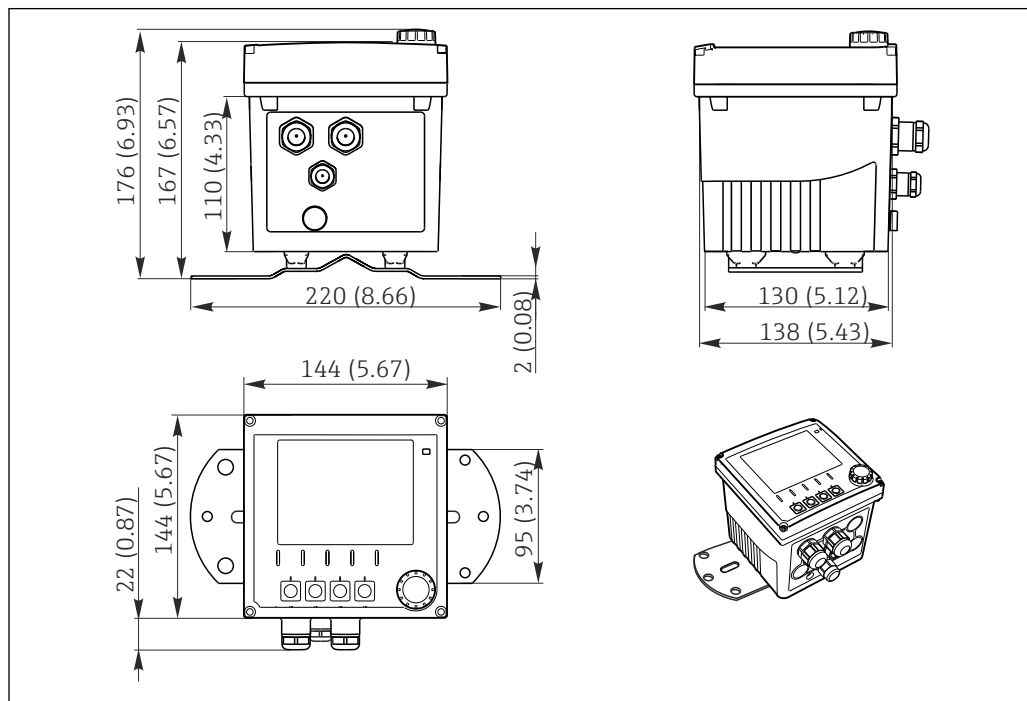
図 59 寸法 (mm (インチ) 単位)
