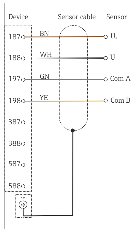
図 25 配線図
