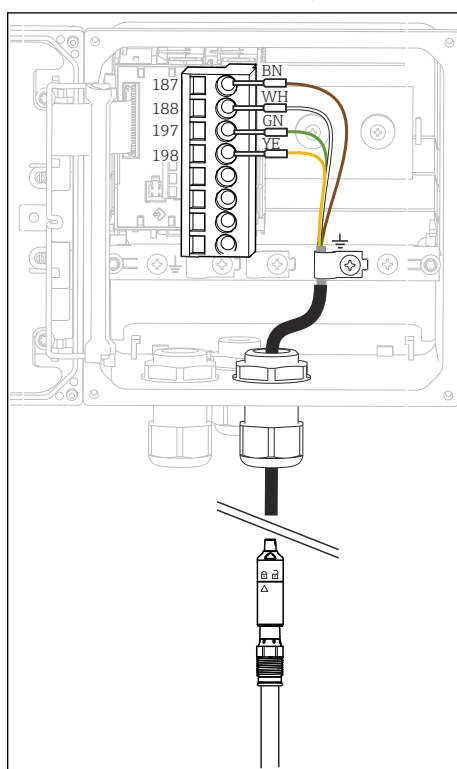
図 22 機器内部図（センサモジュール）
