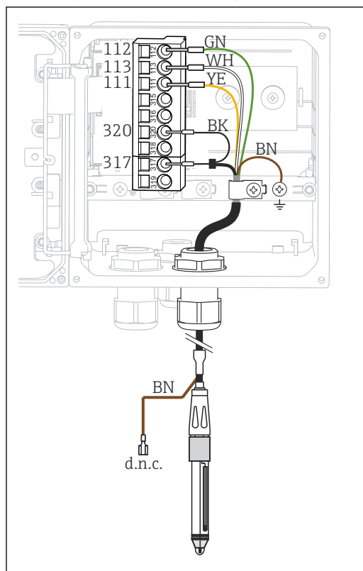
図 28 機器内部図（センサモジュール）
