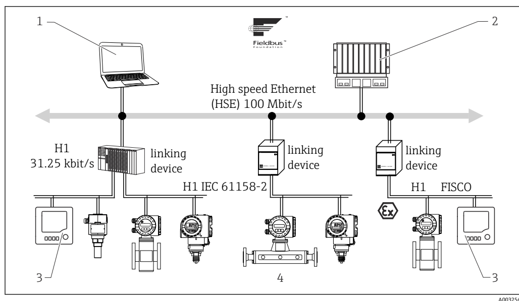
図 66 関連コンポーネントを含むシステム構造
