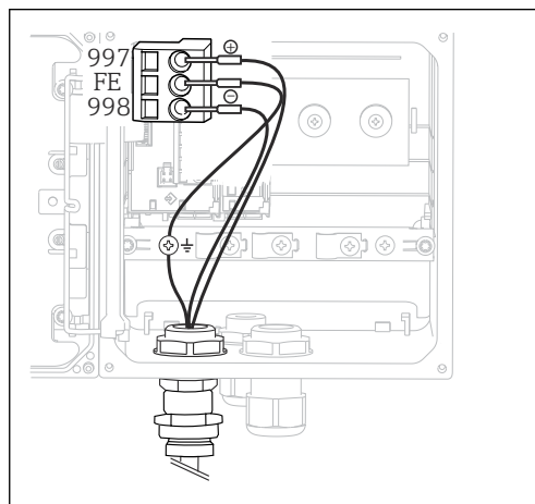
図 20 機器内部図 (CPU モジュール)
