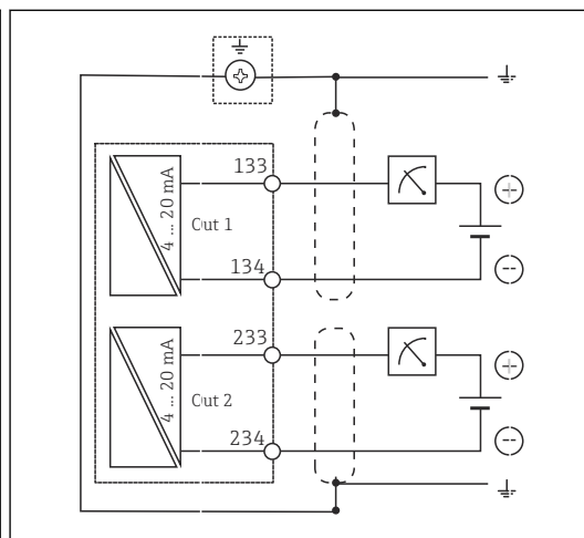
図 15 配線図
