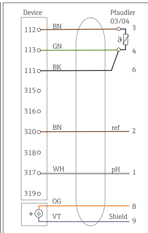
37 配線図
