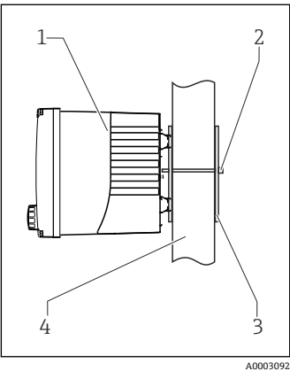
図 57 支柱取付け 1 Liquiline 2, 3 取付プレート (1x アクセサ リ) 4 パイプ/支柱 (円形/角形)
