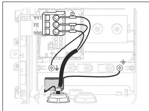
図 18 機器内部図 (CPU モジュール)
