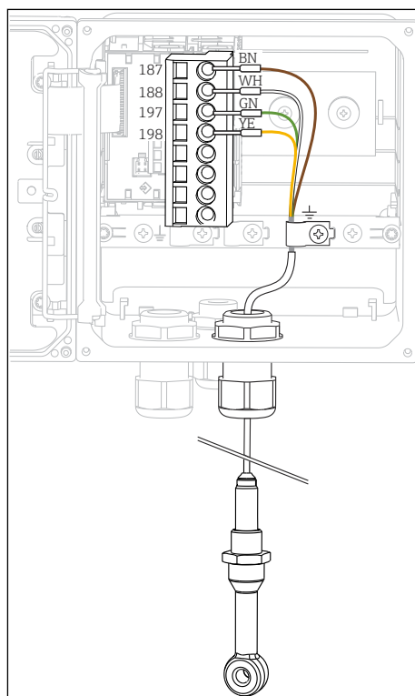
図 24 機器内部図 (センサモジュール)
