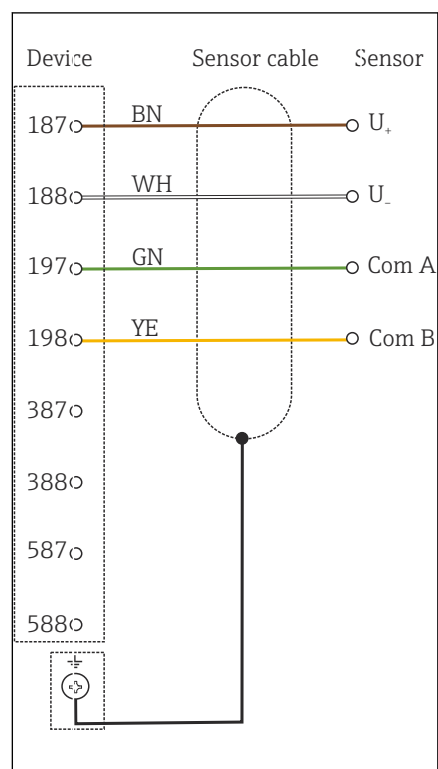
図 23 配線図
