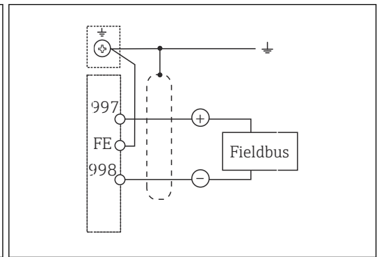
図 17 配線図
