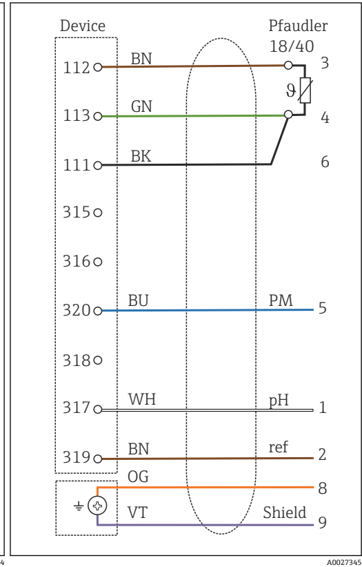
35 配線図
