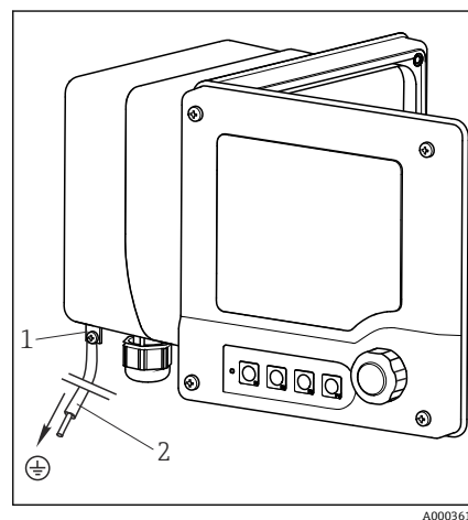
図 11 ハウジングの接地
