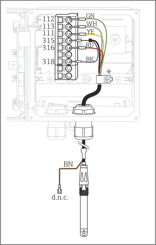
32 機器内部図（センサモジュール）
