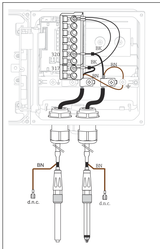
38 機器内部図 (センサモジュール)
