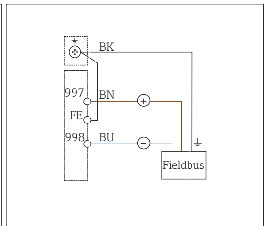
図 21 配線図
