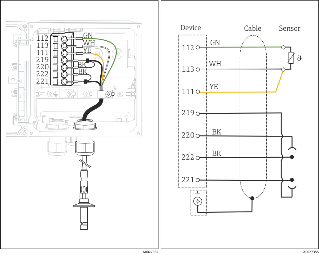
43 機器内部図 (センサモジュール)
