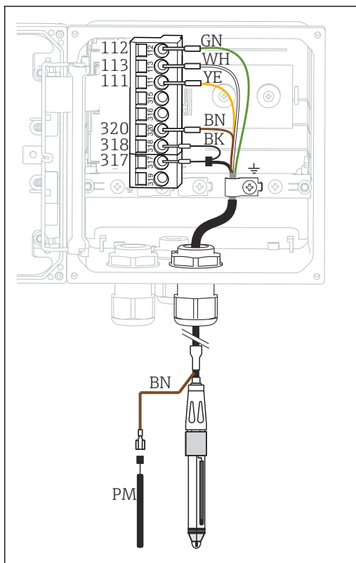
図 26 機器内部図 (センサモジュール)
