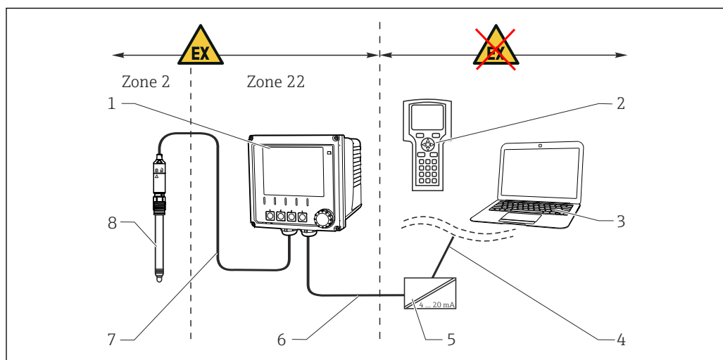
図 52 危険場所 Ex tc (ic) での設置
