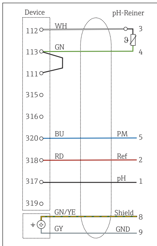
36 配線図
