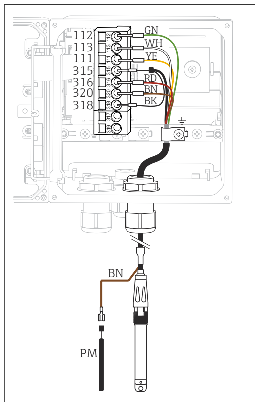
図 30 機器内部図（センサモジュール）
