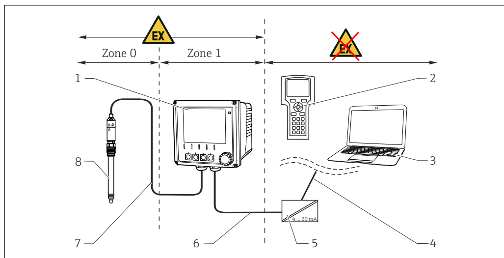
図 51 危険場所 Ex ib (ia Ga) での設置
