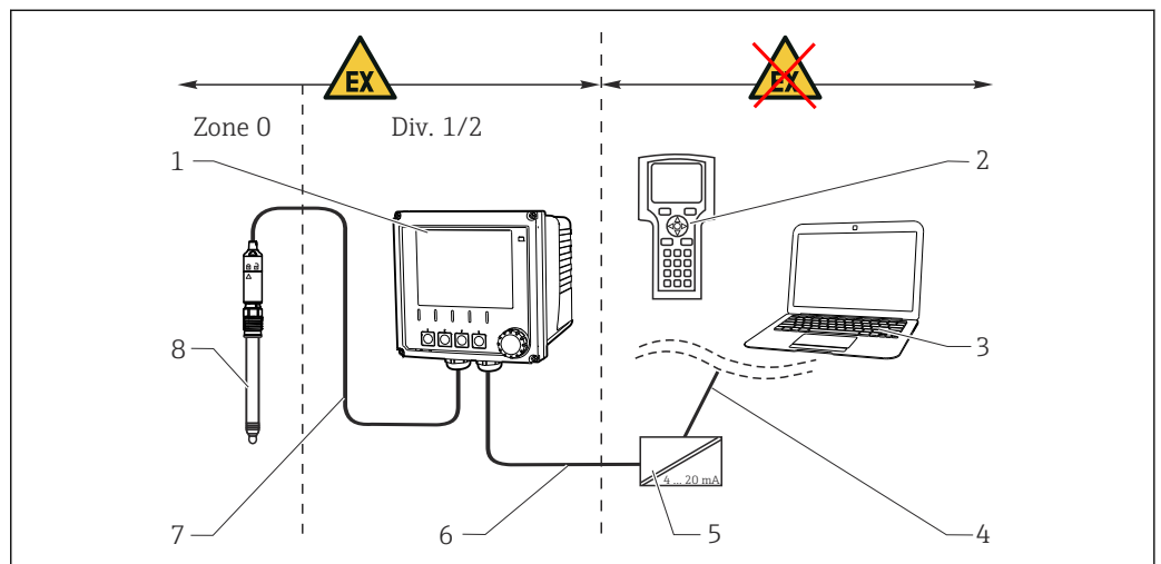
図 54 危険場所 FM/CSA での設置
