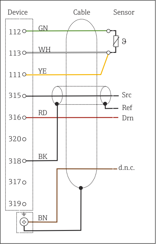
33 配線図
