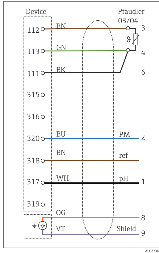
34 配線図
