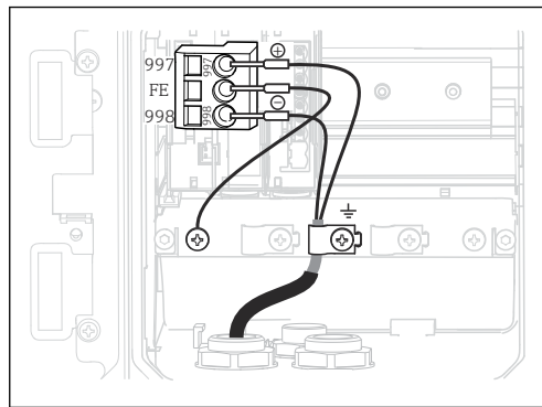
図 16 機器内部図 (CPU モジュール)
