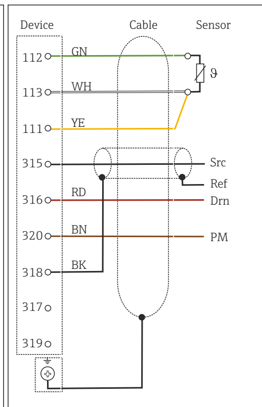
図 31 配線図
