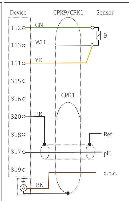
図 29 配線図
