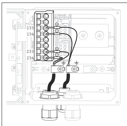
図 12 機器内部図 (CPU モジュール)
