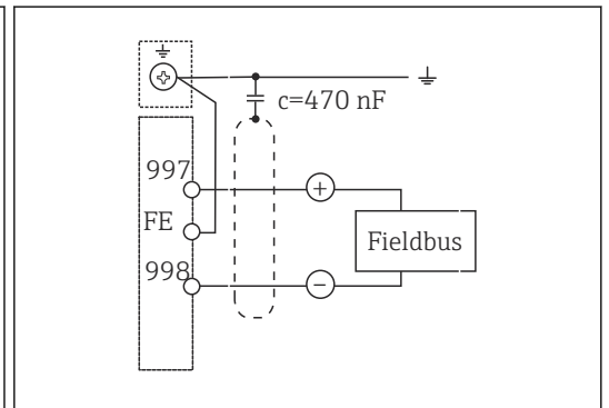
図 19 配線図
