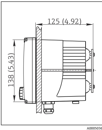
図 58 パネルへの取付け
