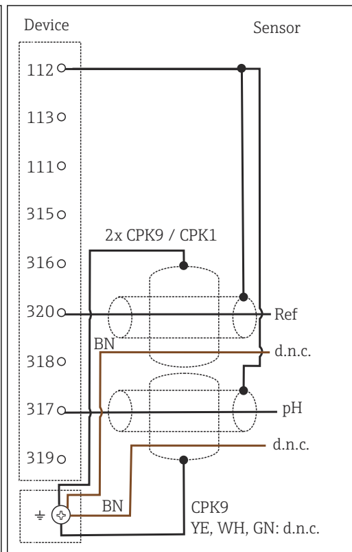
39 配線図
