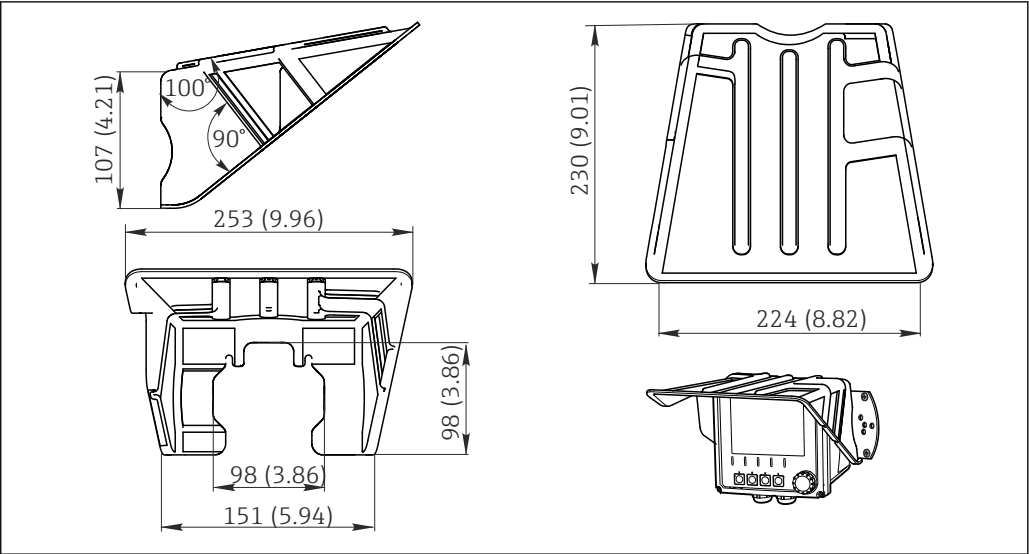
49 寸法 (mm (インチ) 単位)
