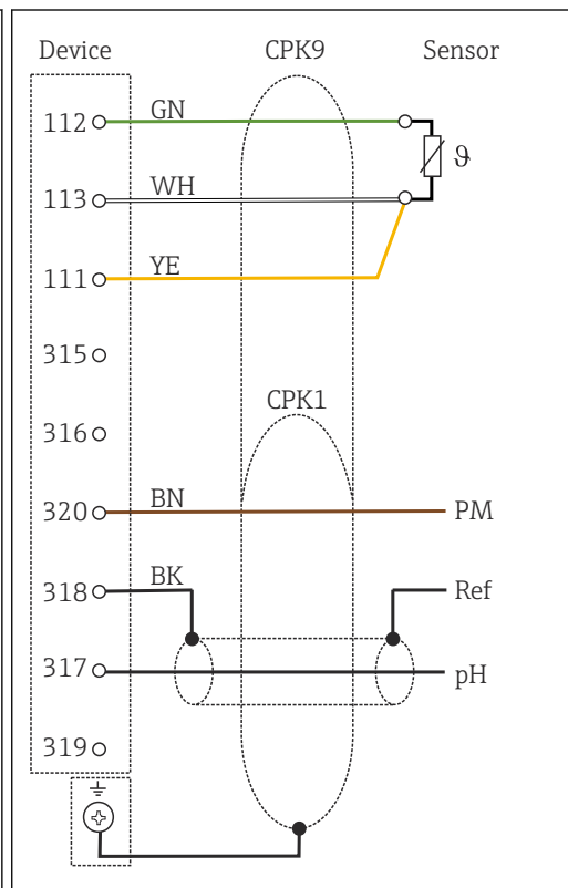
図 27 配線図
