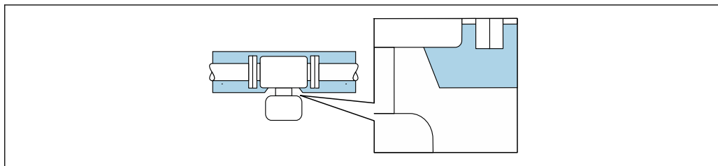
32 Isolation thermique avec tube prolongateur exposé
