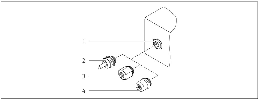
46 Entrées de câble/presse-étoupe possibles
