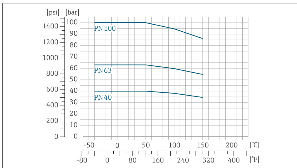
23 Avec matériau de bride 1.4404 (F316/F316L)
