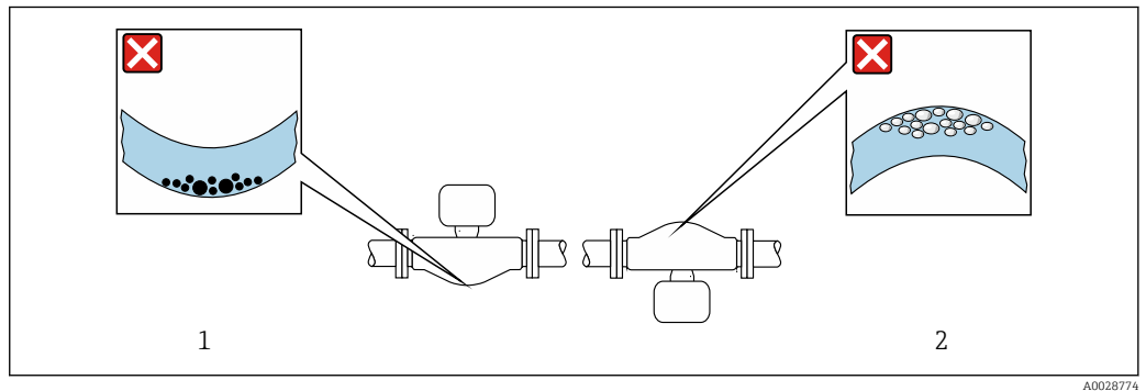
15 Position du capteur avec tube de mesure coudé
