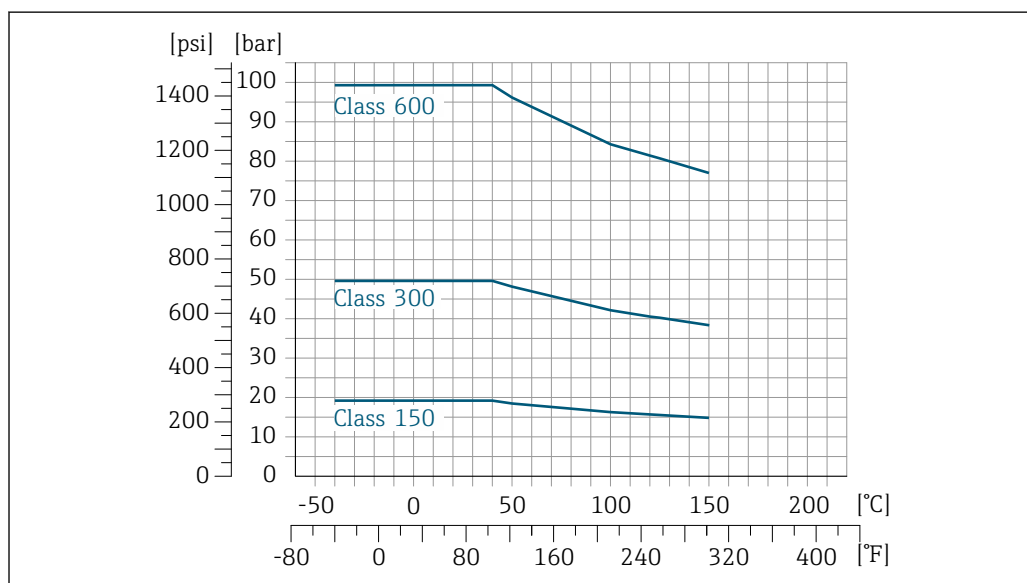
24 Avec matériau de bride 1.4404 (F316/F316L)
