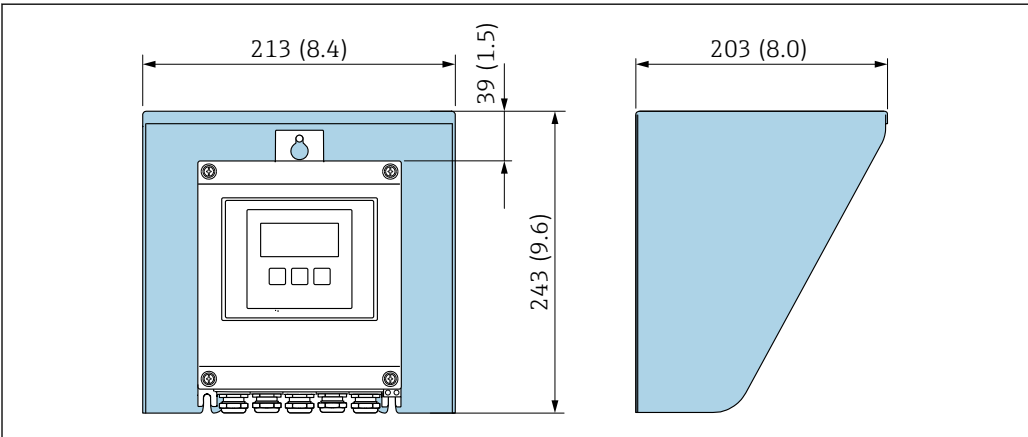
40 Capot de protection climatique pour Proline 500 – numérique ; unité mm (in)
