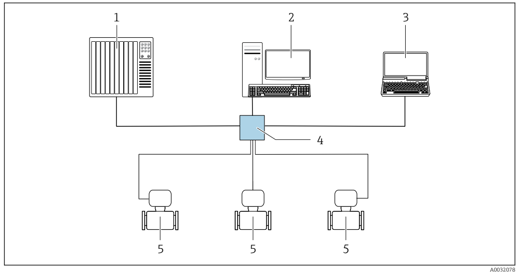
54 Options pour la configuration à distance via le réseau EtherNet/IP : topologie en étoile
