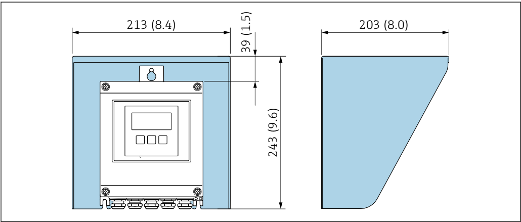
34 Capot de protection climatique pour Proline 500 – numérique ; unité mm (in)
