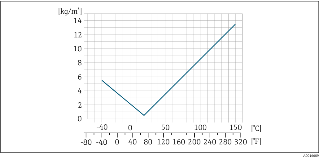
13 Ajustage sur site de la masse volumique, par exemple à +20 °C (+68 °F)
