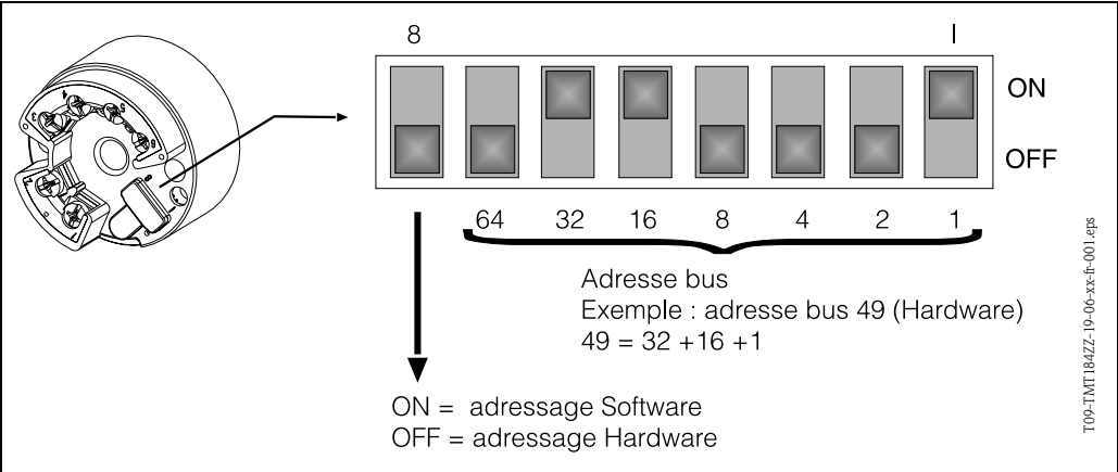
Fig. 6.1: Adressage à l'aide des micro-commutateurs
