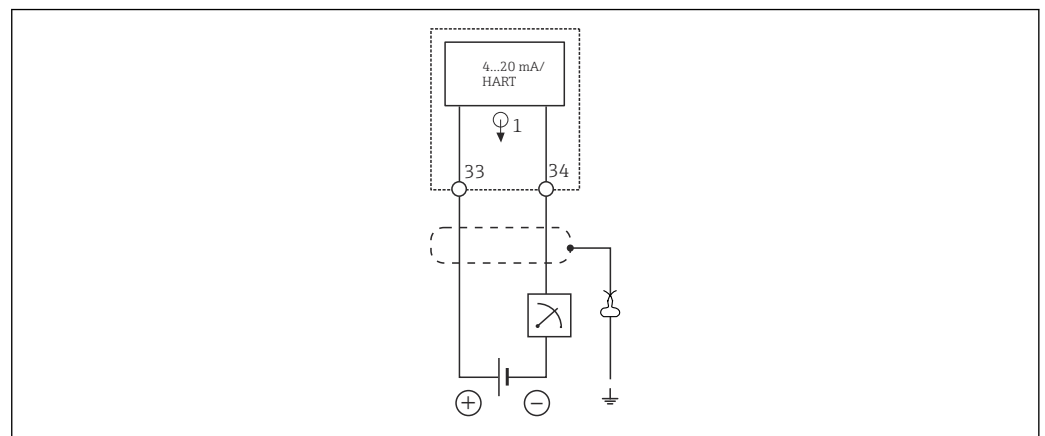
13 Schéma de raccordement : 1 sortie courant (sortie courant avec HART)
