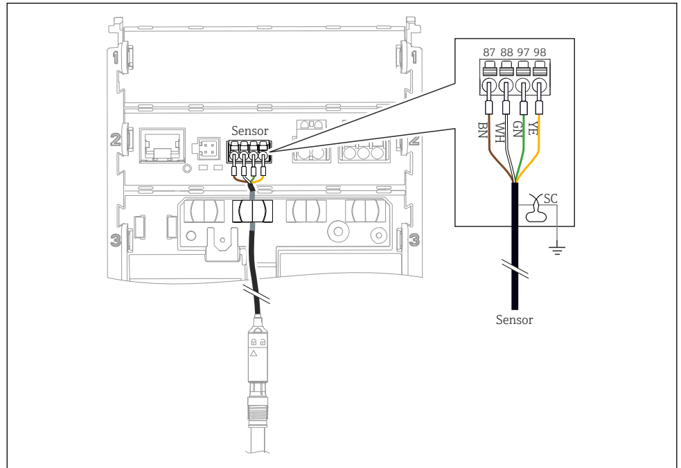
17 Raccordement de capteurs Memosens
