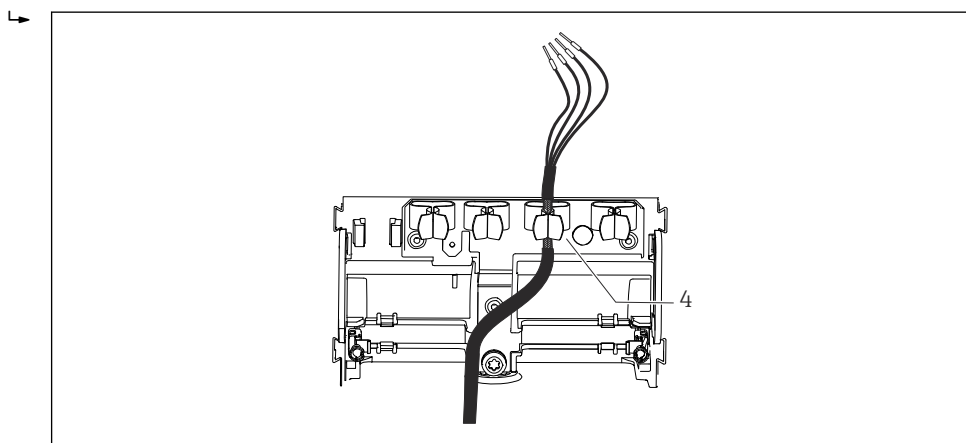
11 Câble dans la bride de mise à la terre
