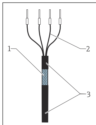
10 Câble préconfectionné
