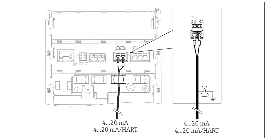
12 Raccordement de 1 sortie courant (exemple: appareil avec HART)
