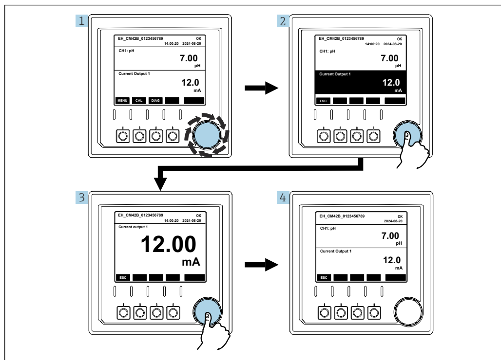
21 Navigation, affichage d'une sortie courant
