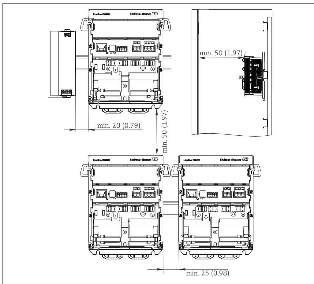
4 Dégagement minimum en mm (in)
