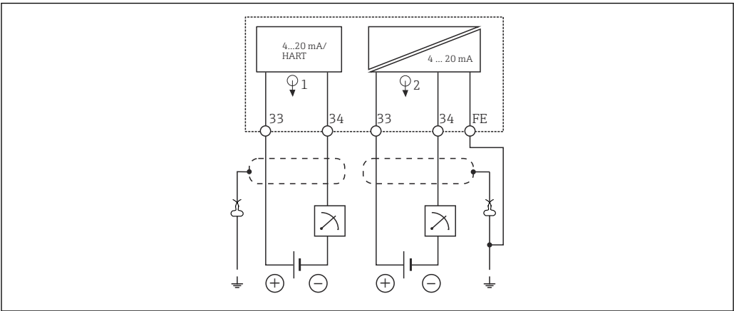
16 Schéma de raccordement : 2 sorties courant (sortie courant 1 avec HART)
