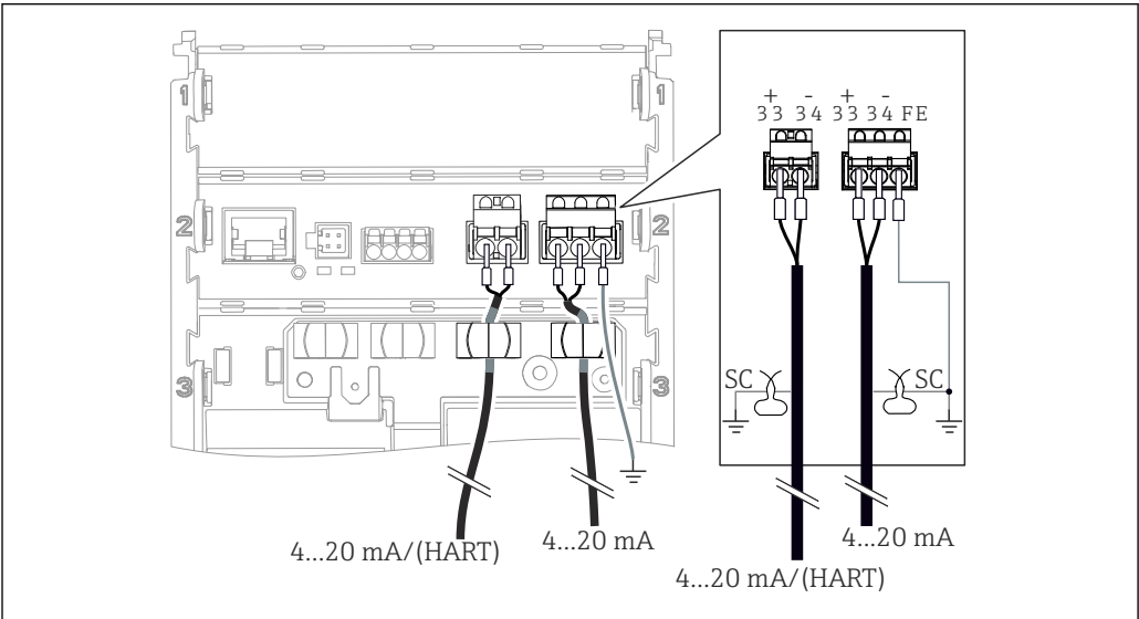
15 Raccordement de 2 sorties courant via 2 câbles blindés (sortie courant 1 avec HART)
