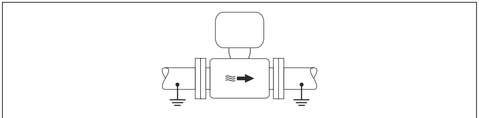
5 Equalizzazione del potenziale mediante il tubo di misura
