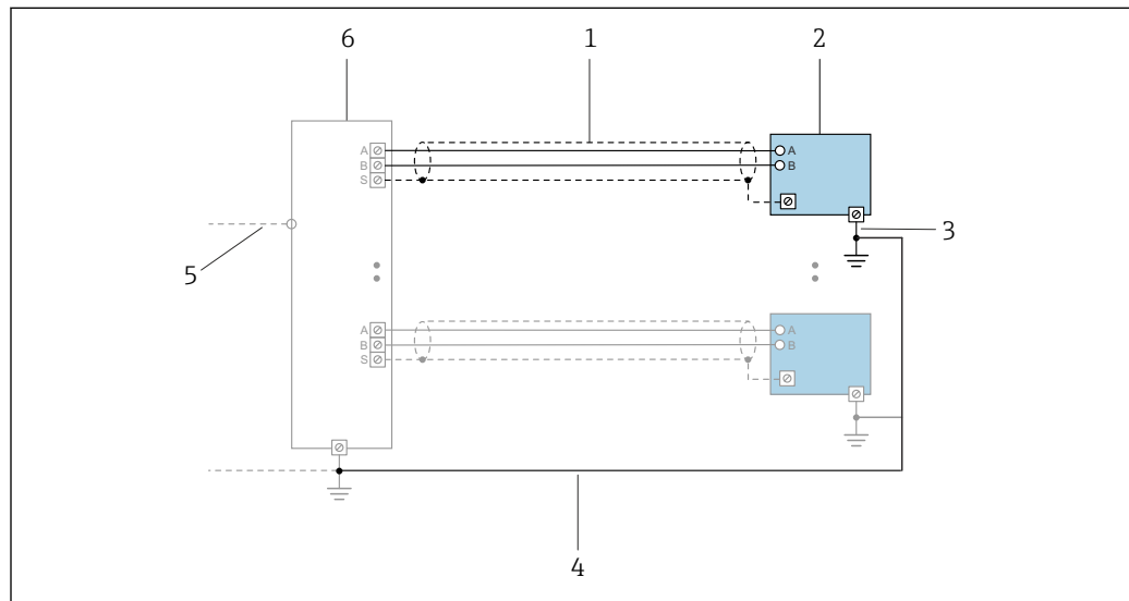
16 Пример подключения для интерфейса PROFINET через Ethernet-APL
