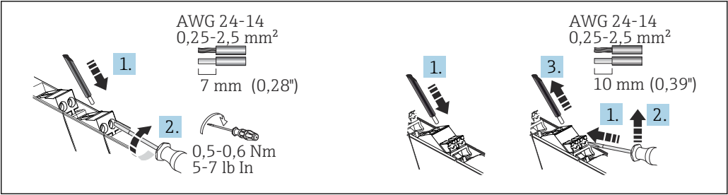
8 Conexão elétrica usando os terminais de parafuso (esquerda) e terminais push-in (direita)
