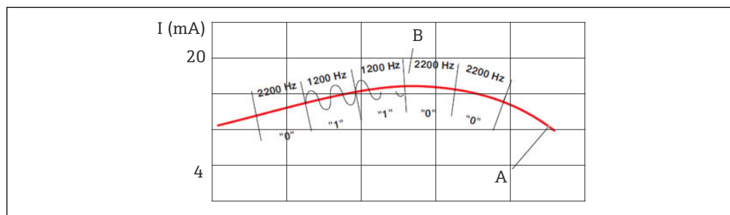
15 Sinal HART modulado
