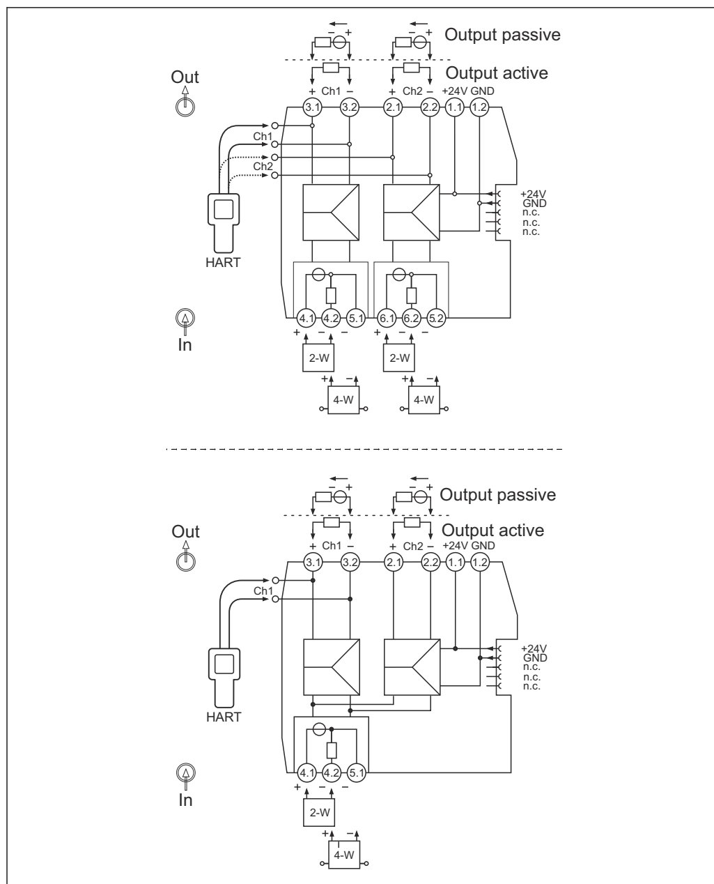
5 Atribuição do terminal: versão com 1 e 2 canais (superior), duplicador de sinal (inferior)
