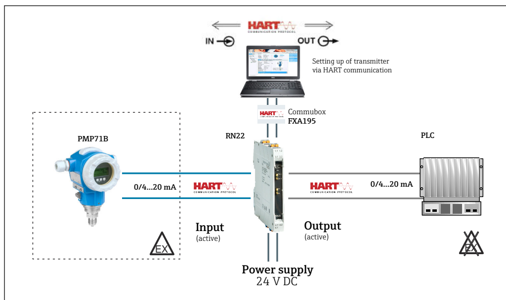
16 Medição de pressão em uma área classificada com uma barreira ativa RN22
