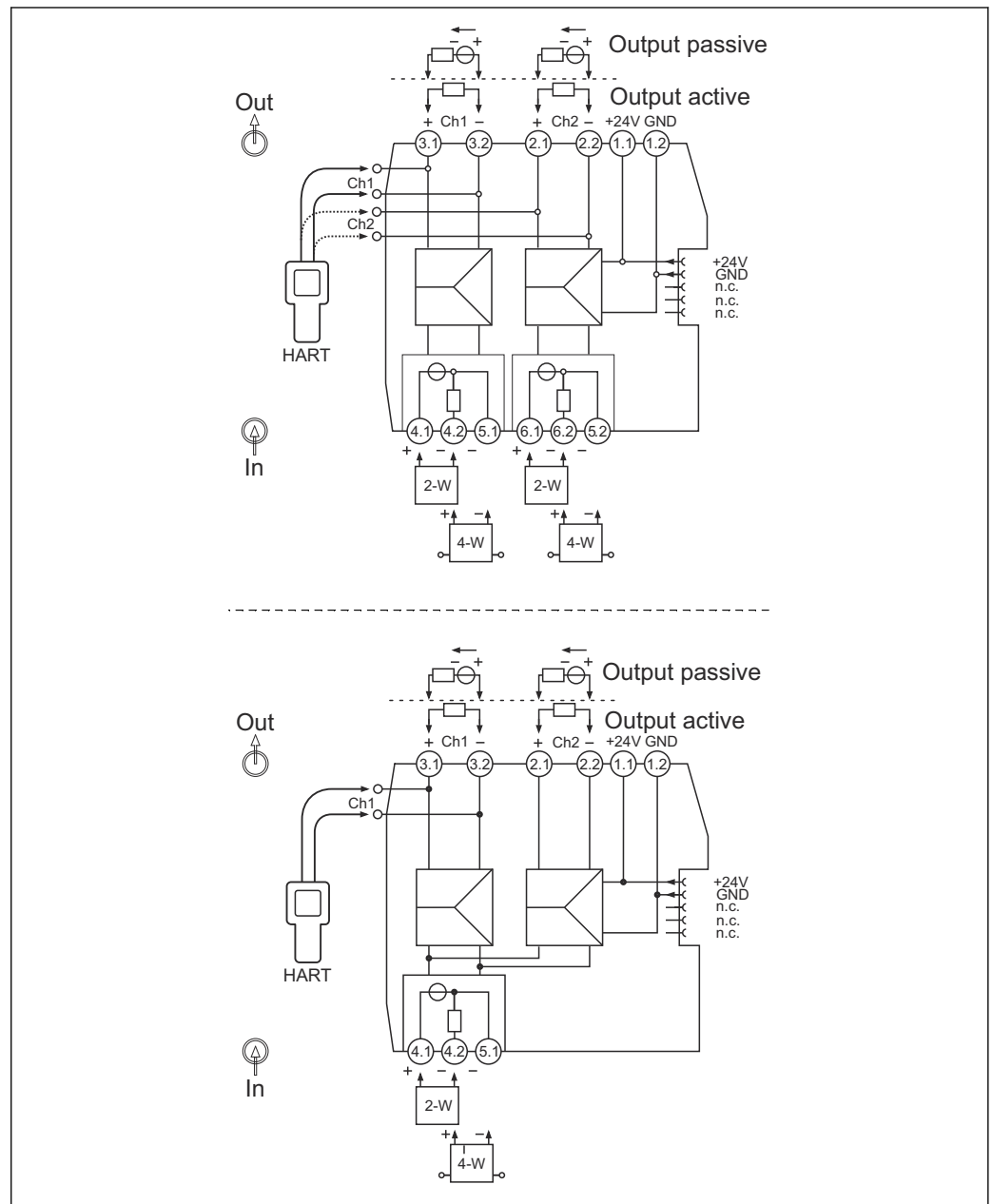
7 Atribuição do terminal: versão com 1 e 2 canais (superior), duplicador de sinal (inferior)
