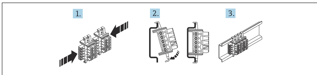
1 Montagem do conector de barramento de trilho DIN 12.5 mm (0.5 in)
