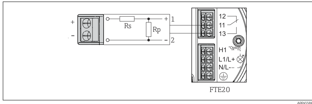
21 Circuito de resistência para monitoramento de linha (curto-circuito e linha aberta)
