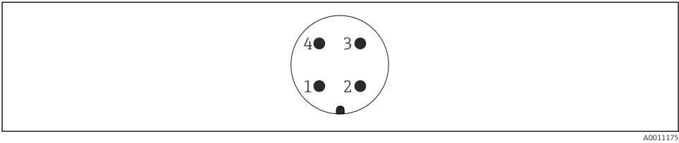
6 M12-pistokkeen napojen kytkennät
