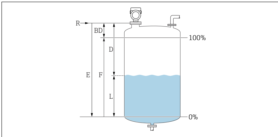
16 Konfigurointiparametrit nesteiden pinnankorkeuden mittaukseen
