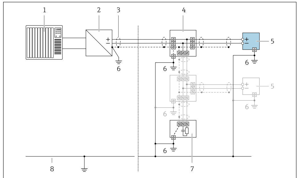
18 Ejemplo de conexión para FOUNDATION Fieldbus
