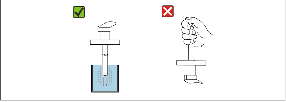
22 Titreşimli çatalın fonksiyonel testi
