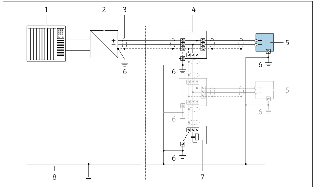
图 18 基金会现场总线(FF)的连接实例
