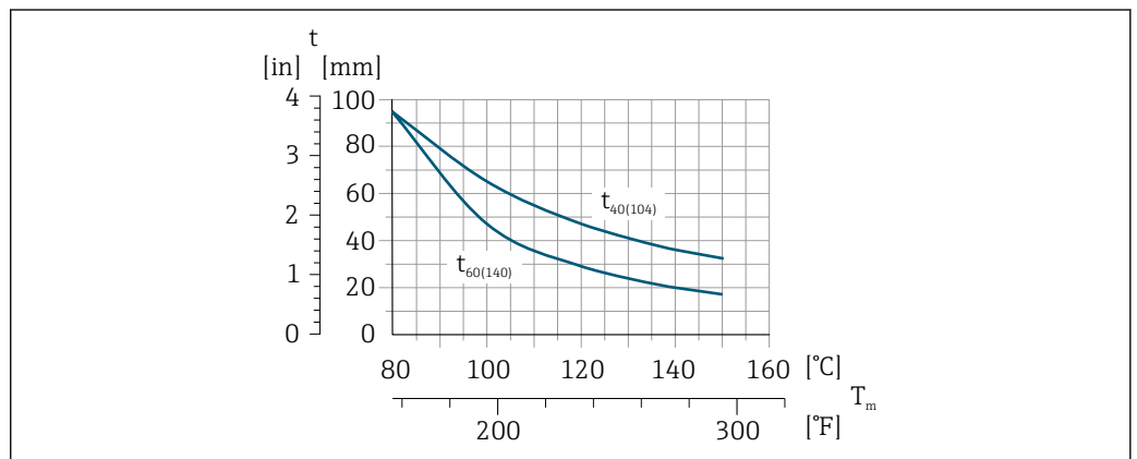
图 9 最大推荐保温层厚度 (t) 取决于介质温度 (T) 和环境温度 ( T_a )
