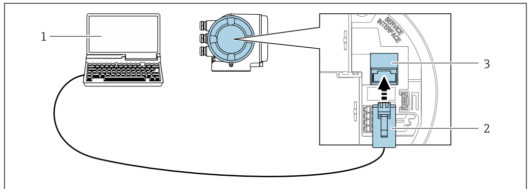
图 30 通过服务接口(CDI-RJ45)操作
