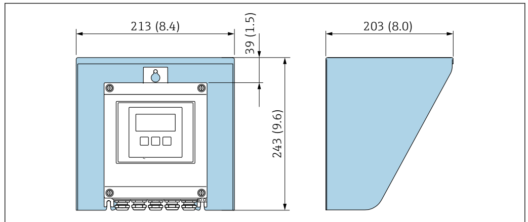
图 10 Proline 500 (数字式)的防护罩
