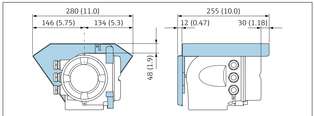
图 11 Proline 500 的防护罩
