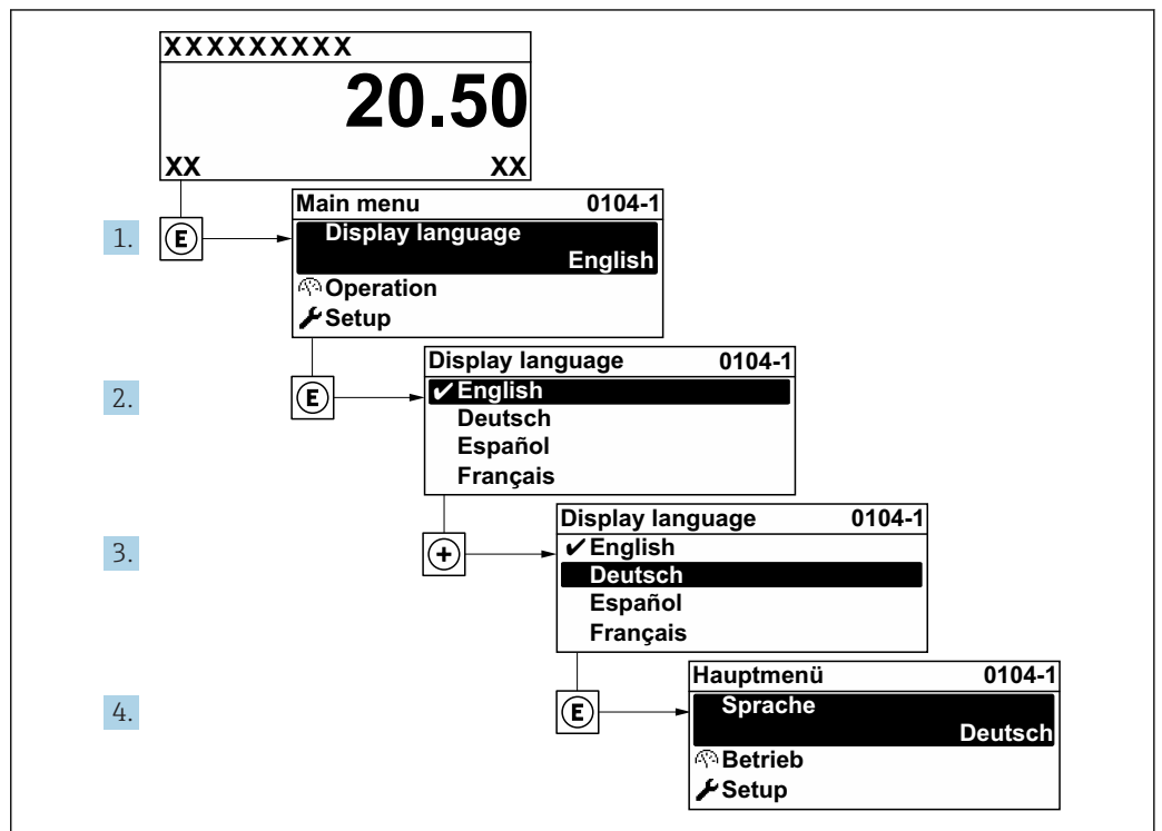
31 现场显示示意图
