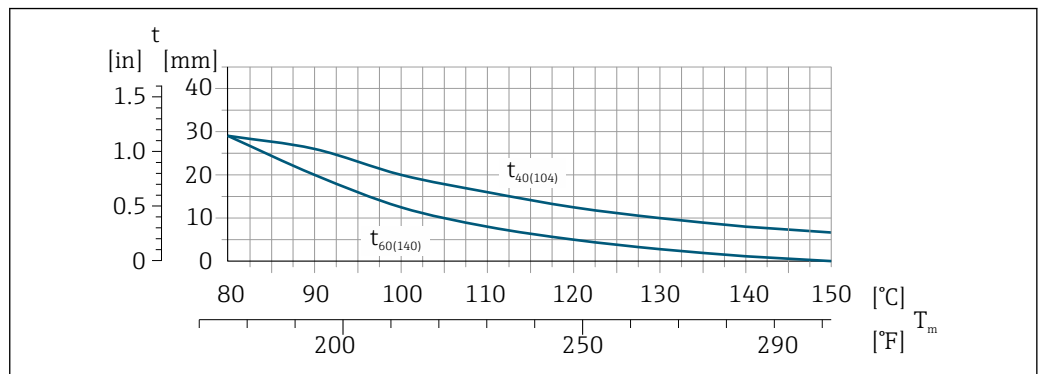
图 8 最大推荐保温层厚度 (t) 取决于介质温度 (T) 和环境温度 ( T_a )
