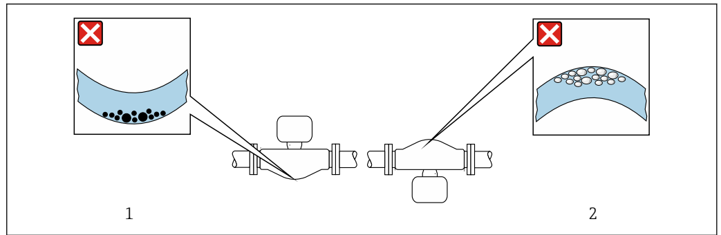
图 7 带弯测量管的传感器的安装方向
