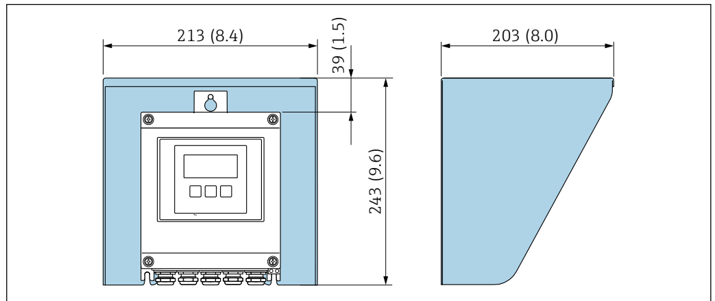
图 9 Proline 500 (数字式)的防护罩
