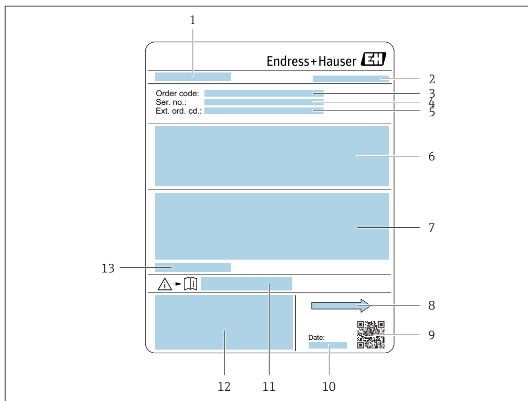
3 Пример заводской таблички сенсора
