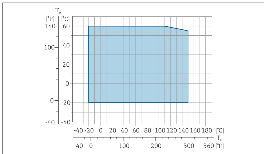
T_a Диапазон температур окружающей среды T_F Температура жидкости
