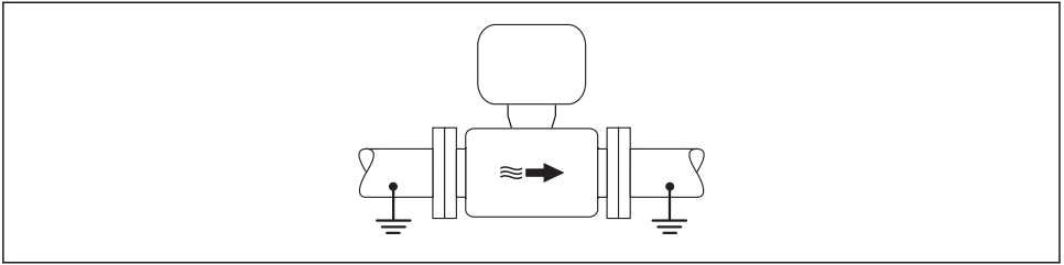
9 Compensation de potentiel via le tube de mesure
