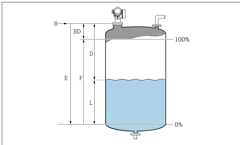
23 Paramètres de configuration pour la mesure de niveau dans les liquides
