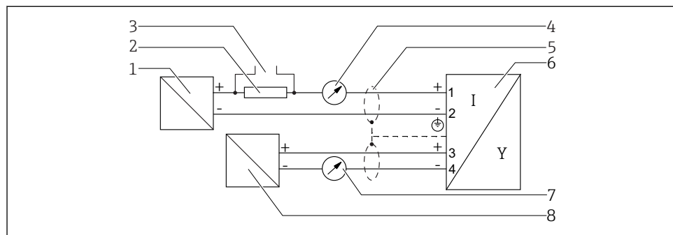
10 Schéma de principe 2 fils : 4-20 mA HART, 4-20 mA
