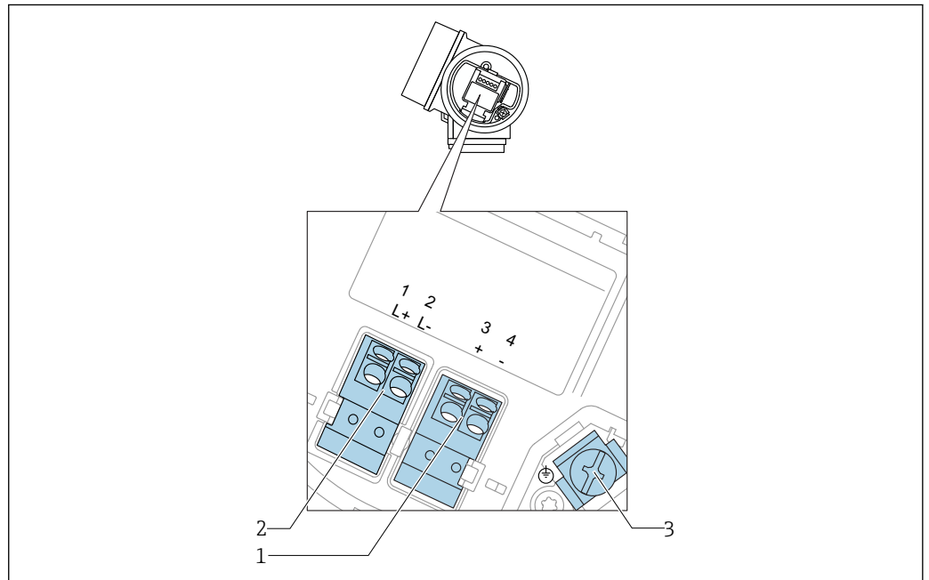
図 16 4 線式、4~20 mA HART の端子割当て (10.4~48 V DC )
