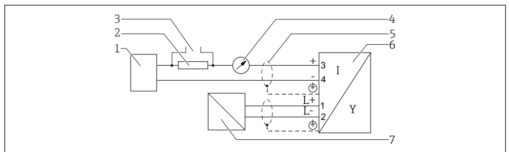
図 17 ブロック図：4 線式、4~20 mA HART (10.4~48 V DC )
