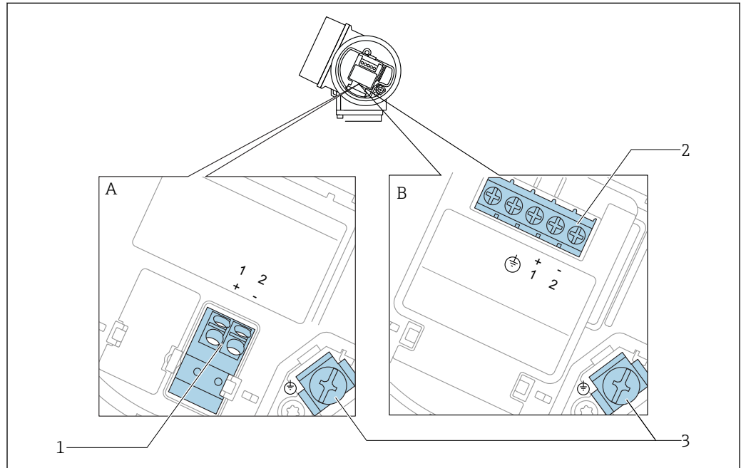
図 10 2線式、4-20 mA HART の端子割当て
