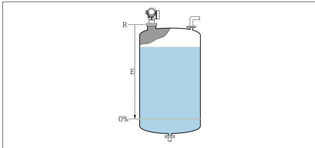
44 液体レベル測定用の空校正 (E)
