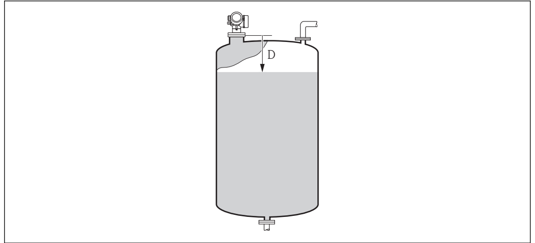
図 47 液体計測の距離
