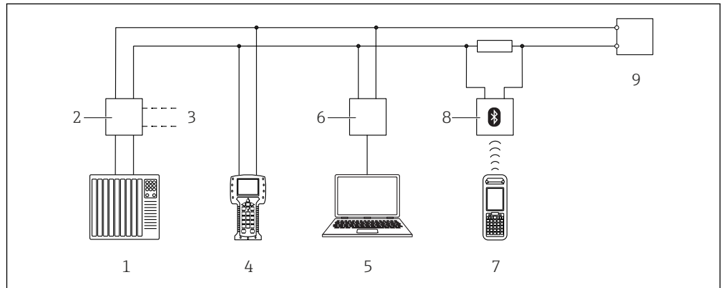
図 27 HART 経由のリモート操作オプション
