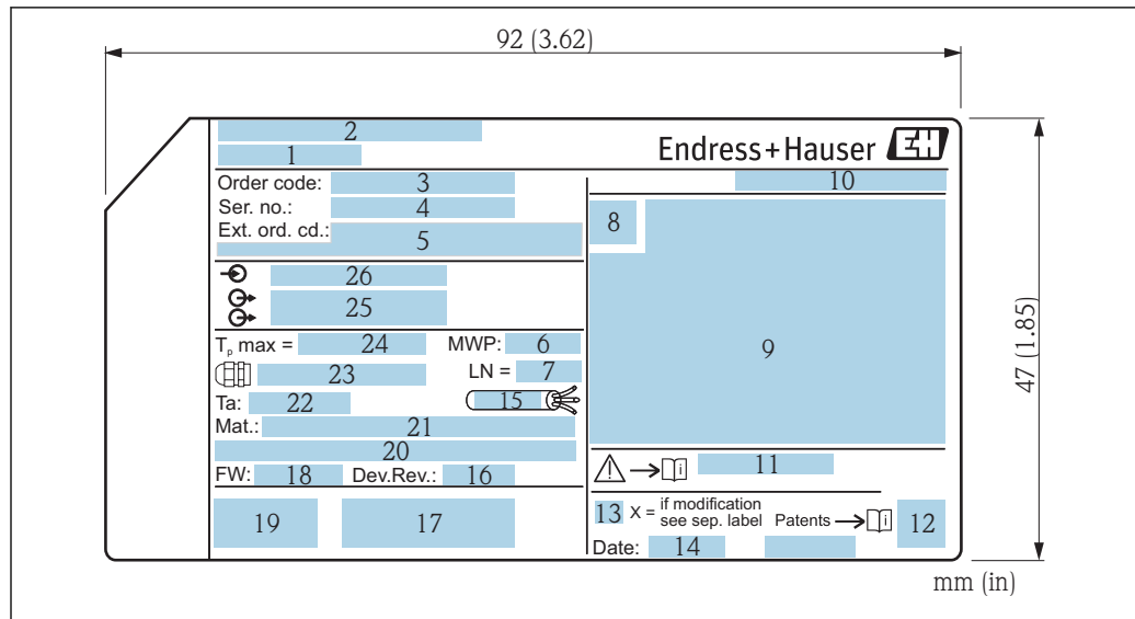
図 4 Micropilot の銘板
