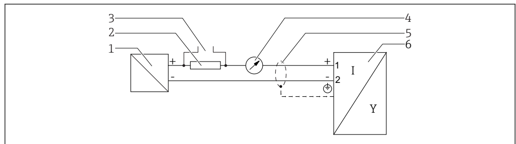
図 11 ブロック図：2線式、4~20 mA HART
