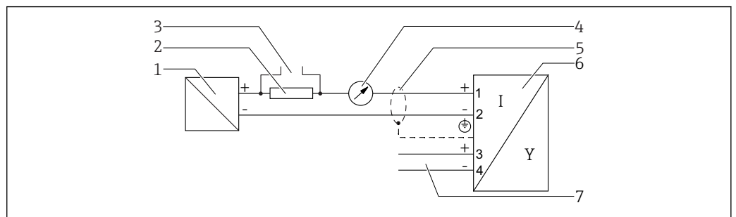
図 13 ブロック図：2線式、4~20 mA HART、スイッチ出力
