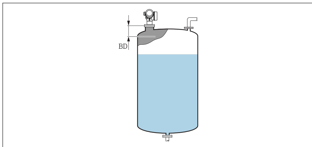
図 52 液体計測の不感知距離 (BD)
