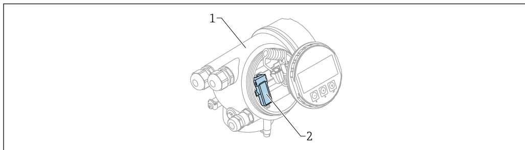
図 25 Bluetooth モジュール搭載の機器
