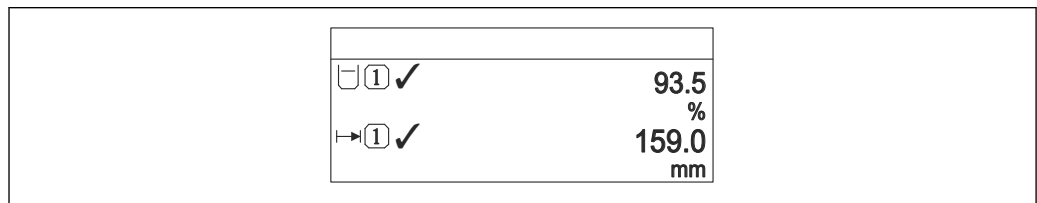
図 55 「表示形式」 = 「2つの値」
