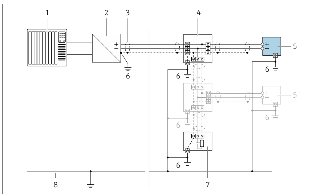
8 Przykład podłączenia wersji z interfejsem FOUNDATION Fieldbus
