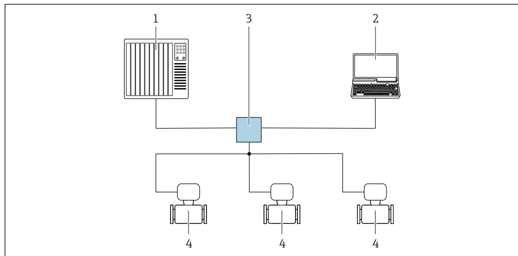
45 Opcje obsługi zdalnej z wykorzystaniem protokołu PROFINET: sieć o topologii gwiazdy
