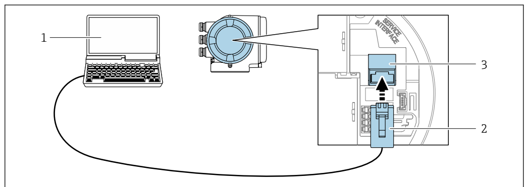
47 Podłączenie poprzez interfejs serwisowy (CDI-RJ45)
