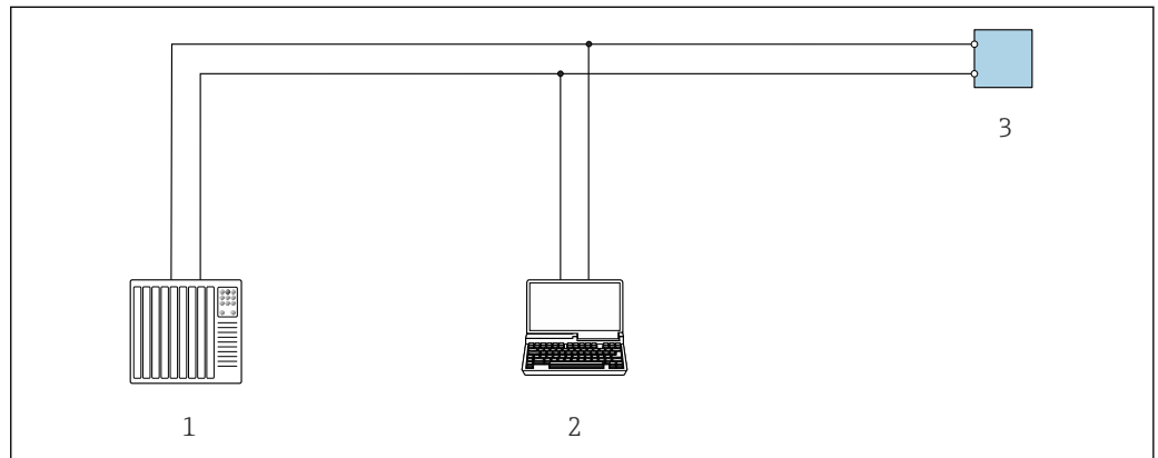
42 Opcje obsługi zdalnej z wykorzystaniem systemu sterowania z wyjściem Modbus-RS485 (aktywnym)
