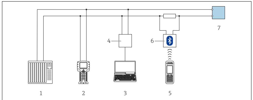
38 Opcje obsługi zdalnej z wykorzystaniem systemu sterowania z wyjściem HART (aktywnym)
