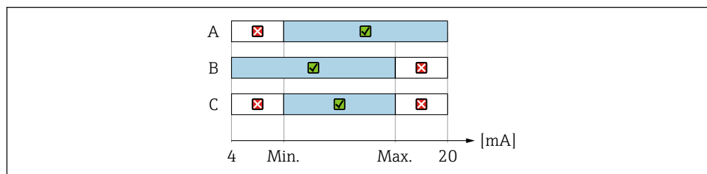
6 Варианты мониторинга в системах защиты
