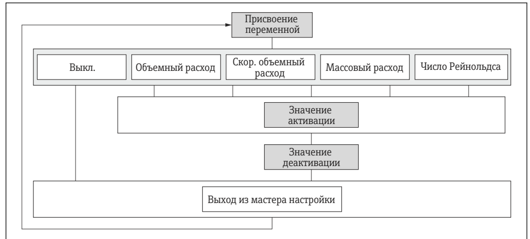
21 Мастер "Отсечение при низком расходе" в разделе меню "Настройка"
