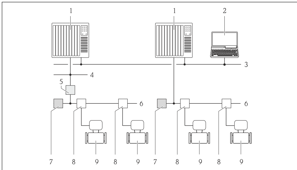
15 Варианты дистанционного управления через сеть FOUNDATION Fieldbus
