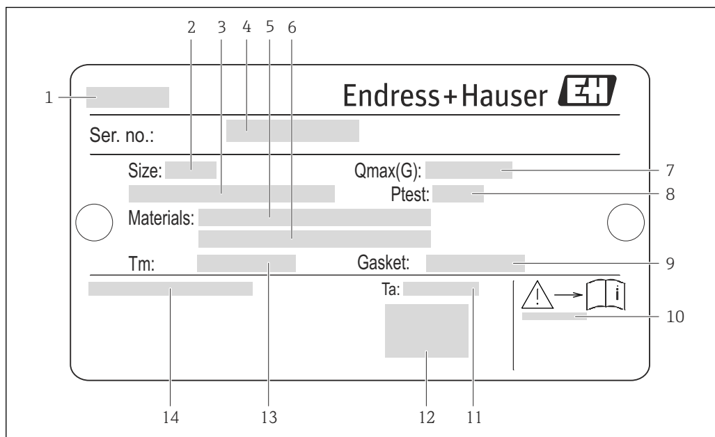
3 Пример паспортной таблички сенсора
