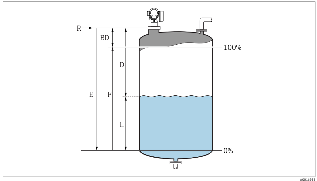
30 Paramètres de configuration pour la mesure de niveau dans les liquides
