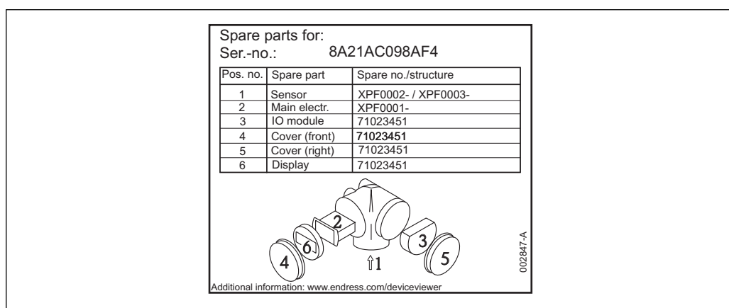
33 Exemple de plaque signalétique dans le couvercle du compartiment de raccordement
