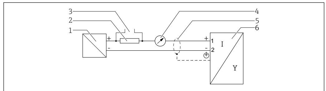
6 Schéma de principe 2 fils : 4-20 mA HART
