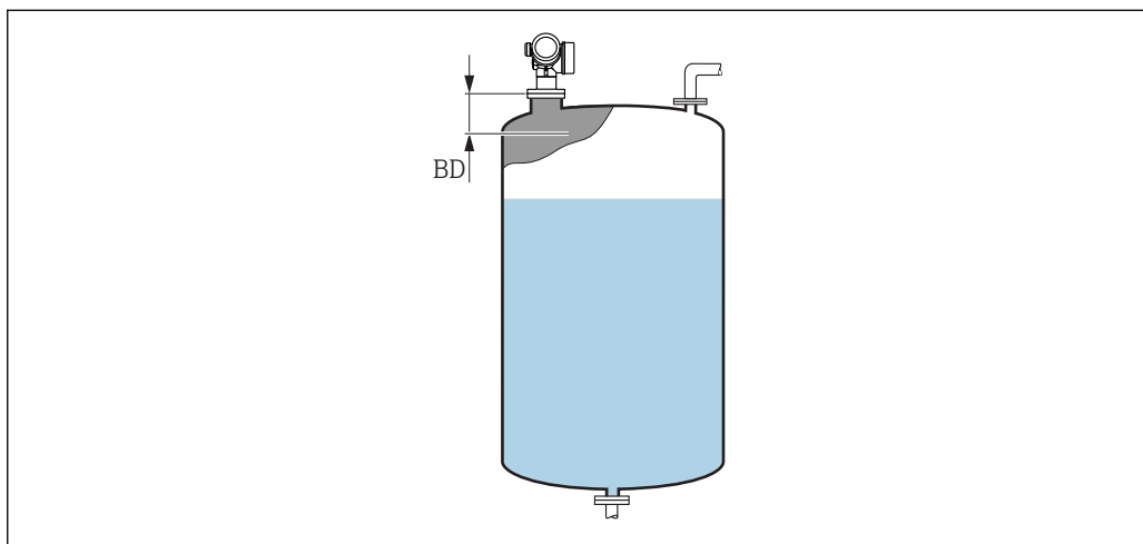
42 Distance de blocage (BD) pour la mesure dans les liquides
