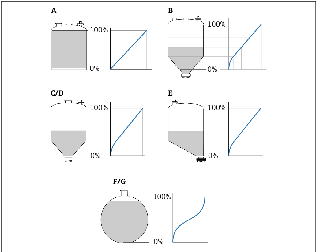
41 Types de linéarisation
