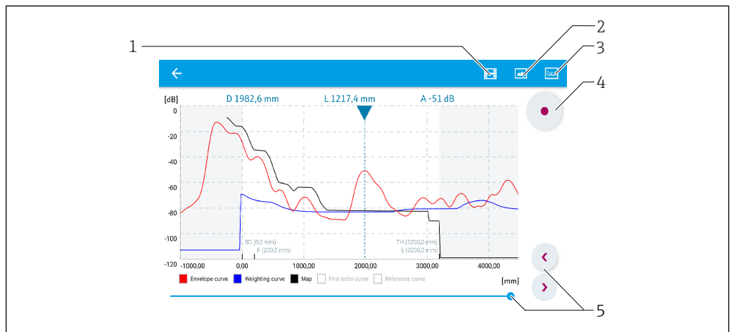
27 Affichage de la courbe enveloppe (exemple) dans SmartBlue ; vue Android
