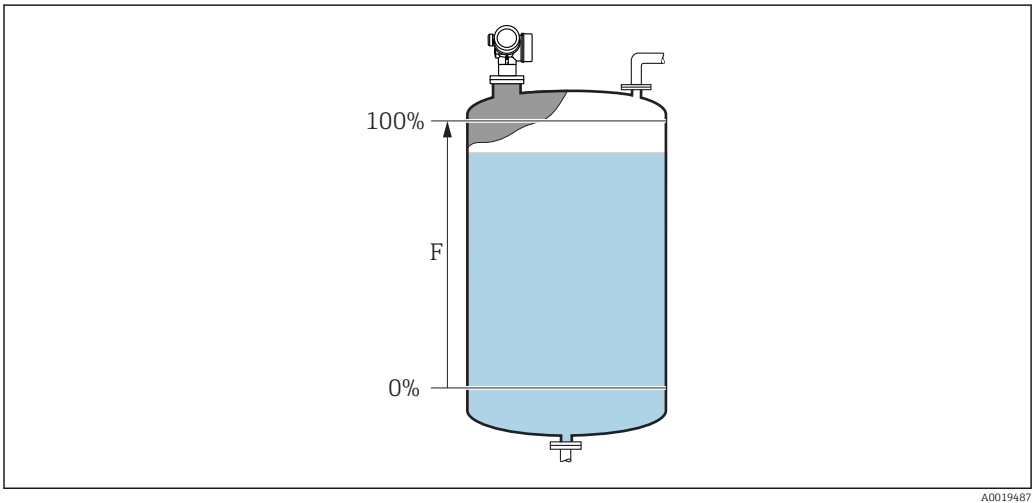
36 Plage de mesure (F) pour la mesure sur liquides
