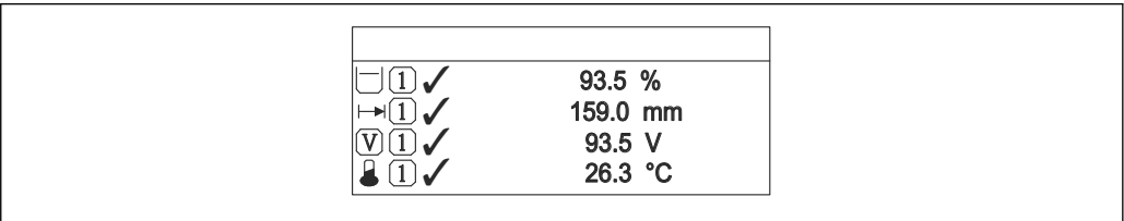
47 "Format d'affichage" = "4 valeurs"
