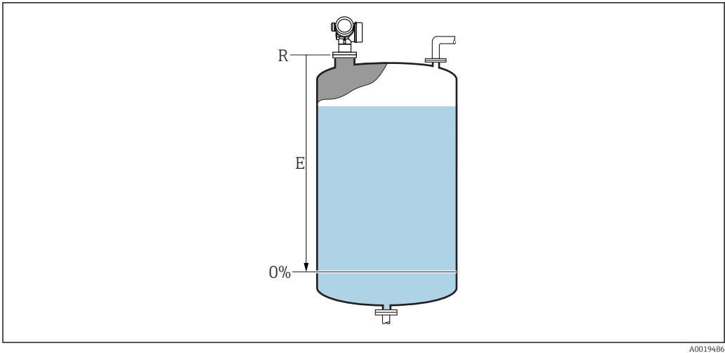
35 Distance du point zéro (E) pour la mesure sur liquides
