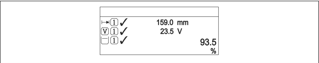
46 "Format d'affichage" = "3 valeurs, 1 grande"
