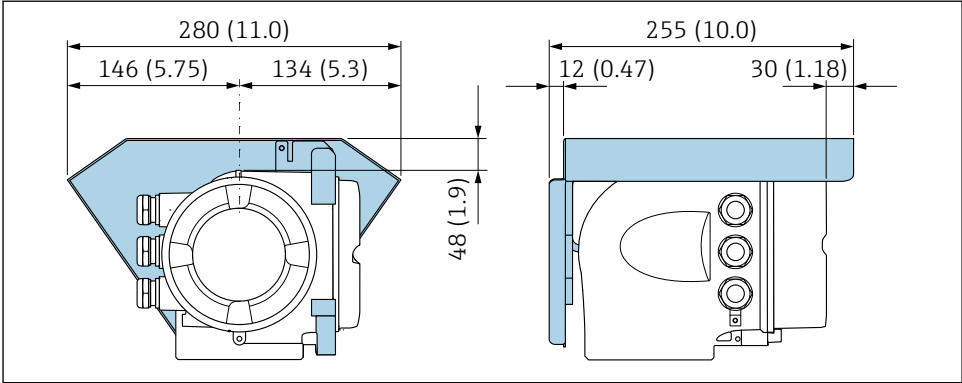
☐ 5 Proline 500용 내후성 커버
