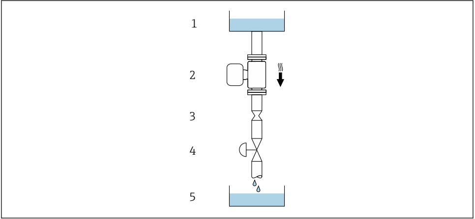
☐ 2 하향 파이프에 설치(예: 배칭 용도)
