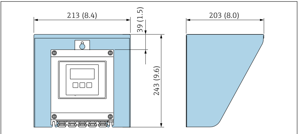
4 Proline 500용 내후성 커버 - 디지털
