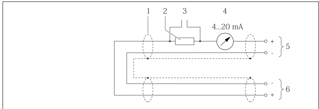
图 17 HART 输入(burst 模式)的连接示例, 通过有源电流输出
