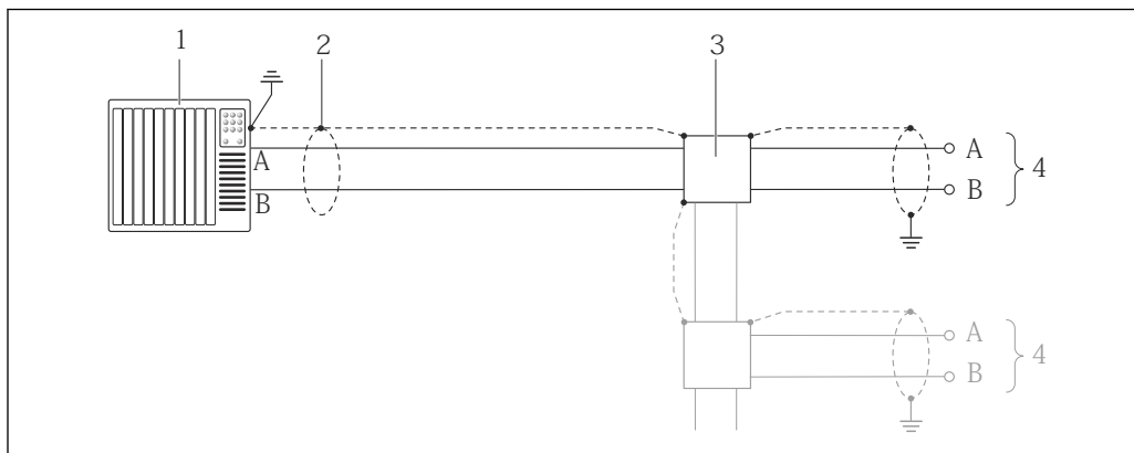
图 13 Modbus RS485 的连接示例，在非危险区和 2 区/ Div. 2 防爆场合中
