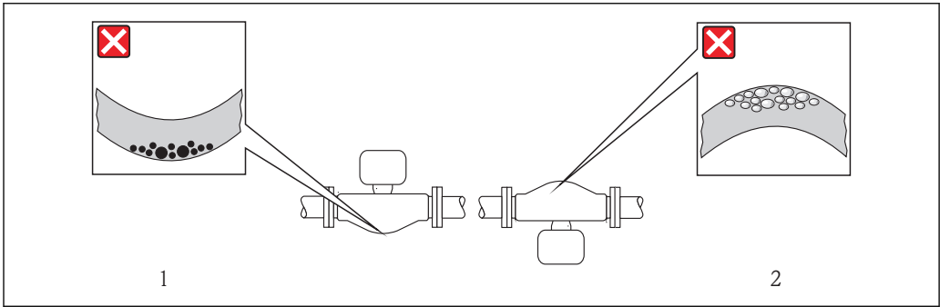
☒ 21 带弯测量管的传感器的安装方向示意图
