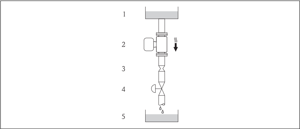
图 20 在向下排空管道中安装(例如：批处理应用)
