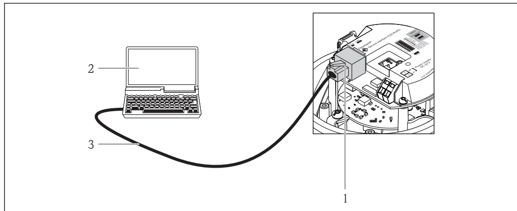
50 订购选项“输出”，选型代号 N: 工业以太网(EtherNet/IP)
