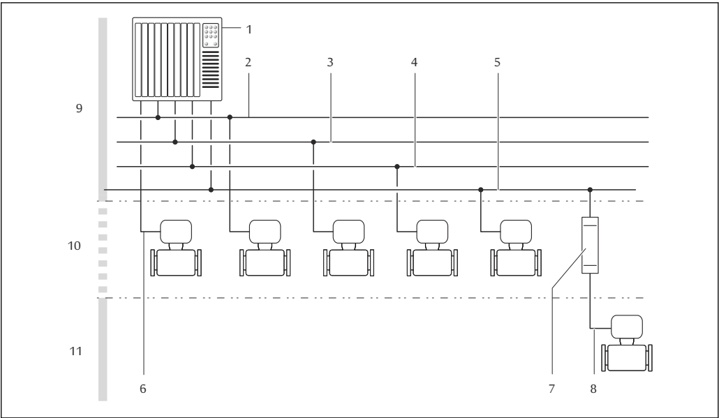
1 测量设备的系统集成示意图
