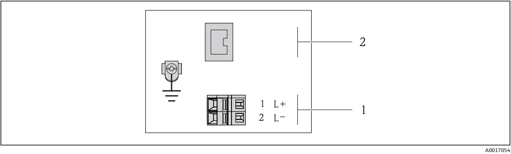
7 PROFINET 接线端子分配示意图
