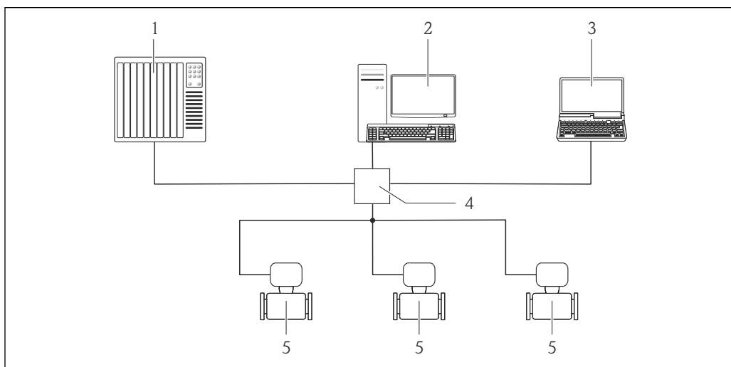
图 46 通过以太网现场总线进行远程操作
