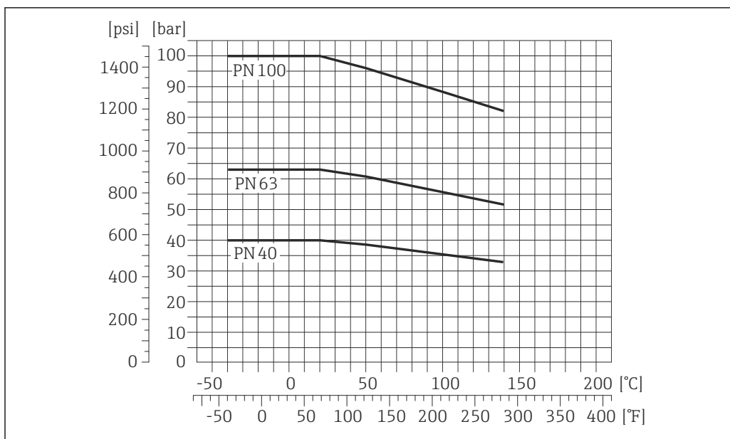
24 法兰材料: 1.4404 (F316/F316L)
