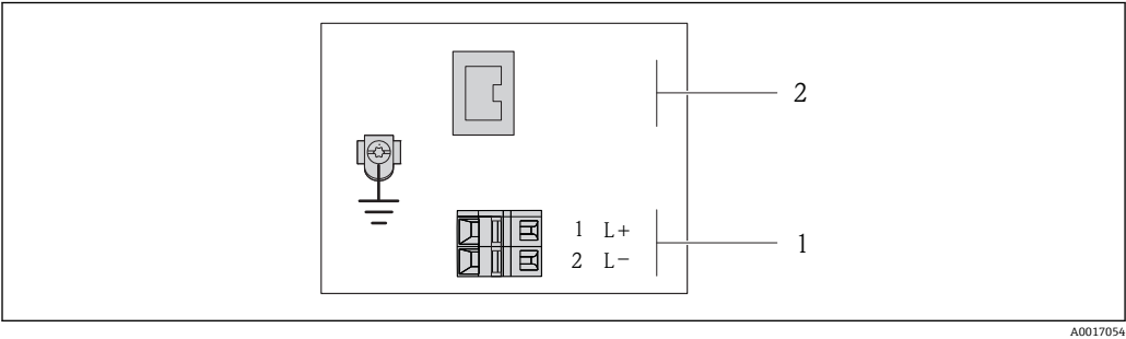
图 6 工业以太网(EtherNet/IP)型仪表的接线端子分配示意图
