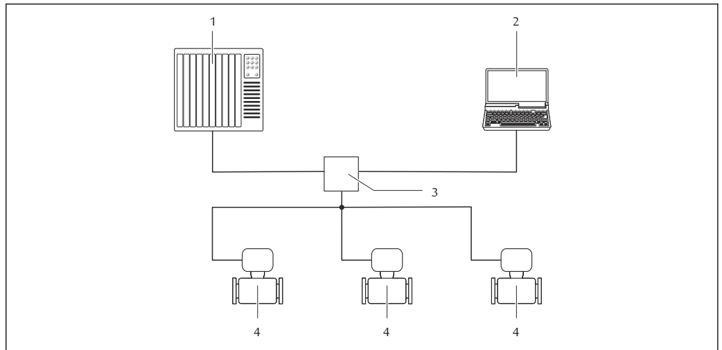
图 47 通过 PROFINET 网络进行远程操作
