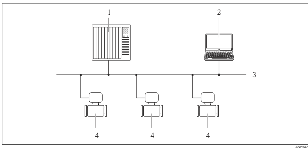
图 45 通过 PROFIBUS DP 网络进行远程操作
