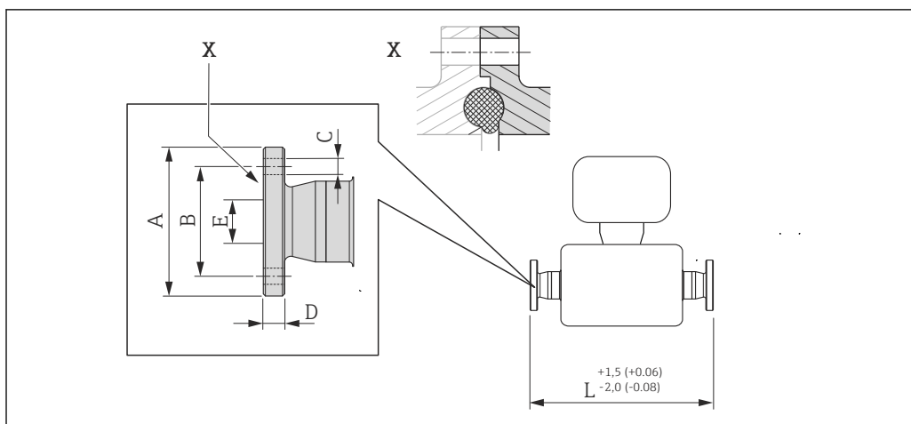
图 34 视图 X: 非对称过程连接; 灰色部分由供应商提供。单位: mm (in)
