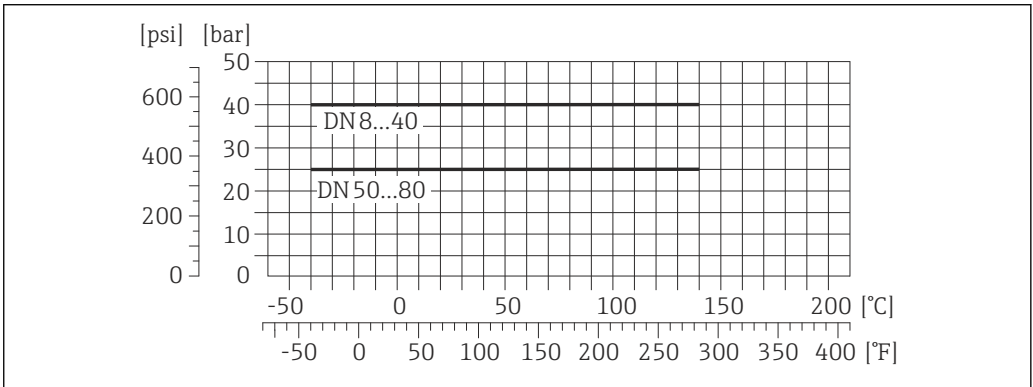
28 连接部件材料: 1.4404 (316/316L)
