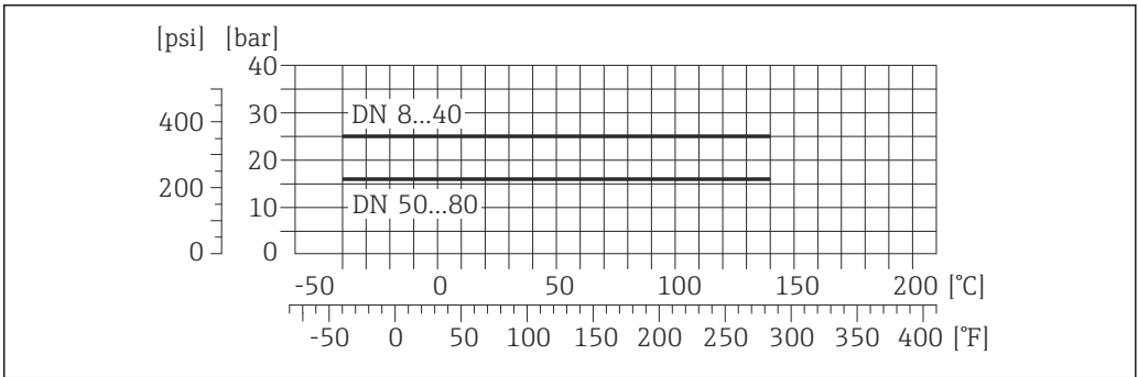
27 法兰材料: 1.4404 (316/316L)
