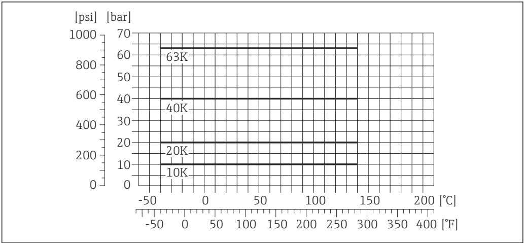
26 法兰材料: 1.4404 (F316/F316L)
