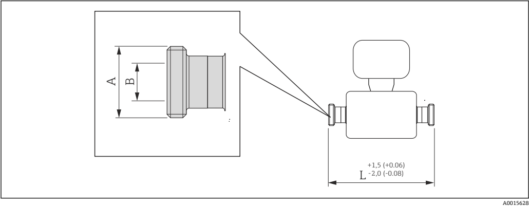
图 36 单位: mm (in)
