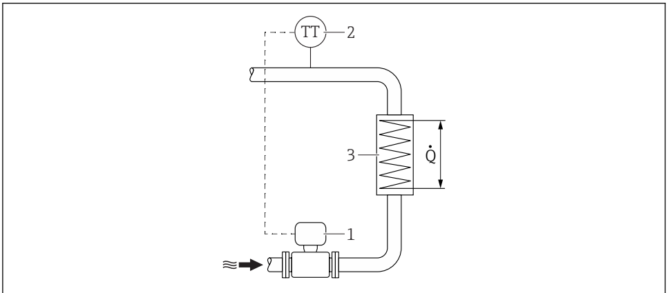
3 Aufbau zur Wärmedifferenzmessung von Satteldampf und Wasser
