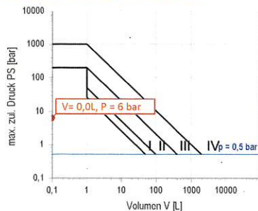
Diagramm 1, Art. 4, Anhang II Behälter, Fluid: Gas, Fluidgruppe: 1 (gefährlich)
