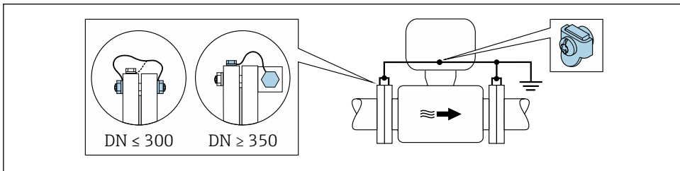
4 Potentiaalın tasaus maadoitusliittimen ja putkilaippojen kautta
