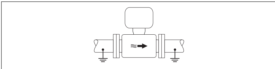
3 Potentiaalın tasaus mittausputken kautta
