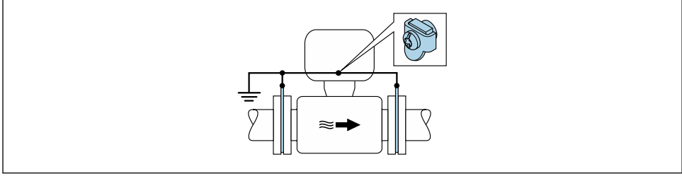
6 Topraklama terminali ve topraklama diskleriyle potansiyel eşitleme
