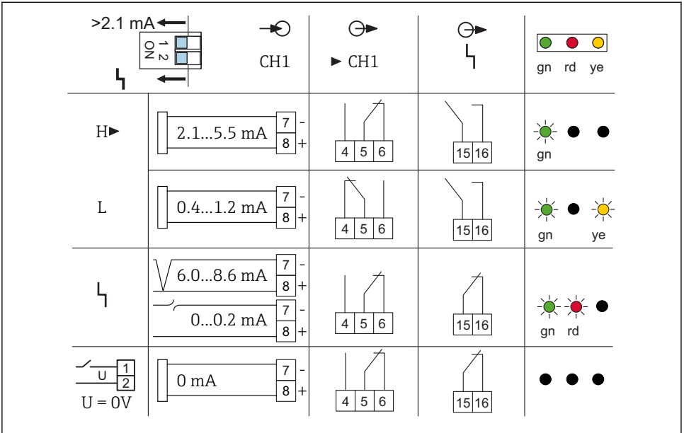
14 Grenzsinal H mit Störungsmeldung (FEL56)
