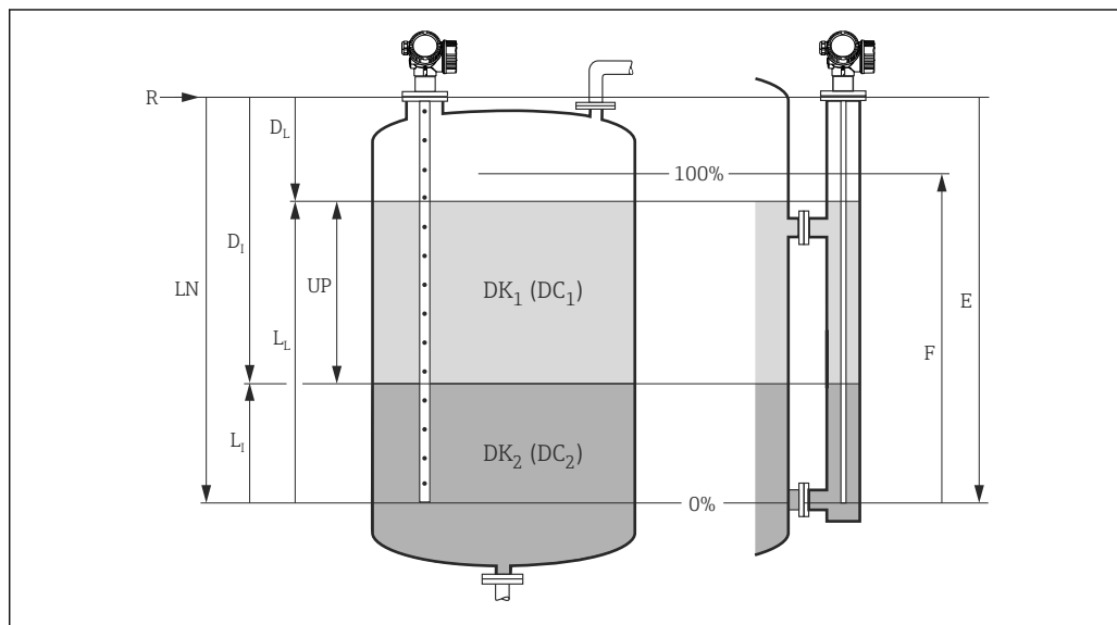
17 Параметры конфигурации измерения уровня границы раздела фаз
