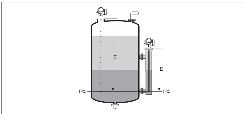
25 Калибровка пустой емкости (E) для измерения уровня границы раздела фаз
