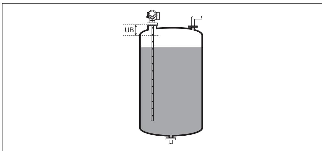
32 Блокирующая дистанция (UB) для измерения в жидких средах
