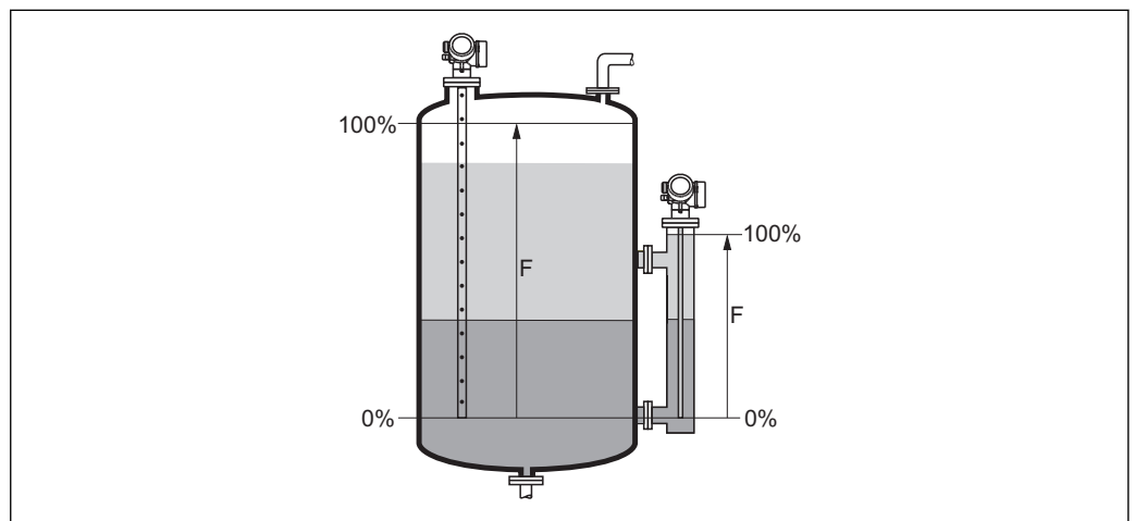
27 Калибровка полной емкости (F) для измерения уровня границы раздела фаз
