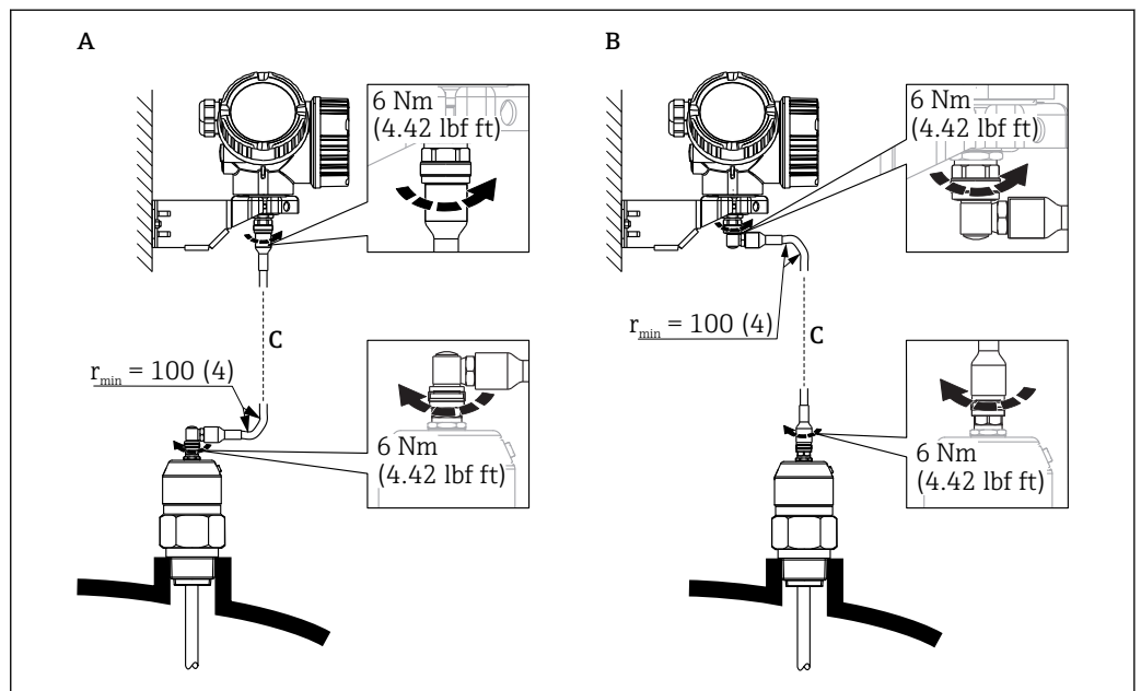
10 Подключение кабеля. Варианты
