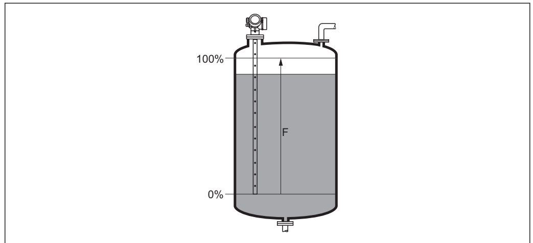
26 Калибровка полной емкости (F) для измерения уровня жидких сред
