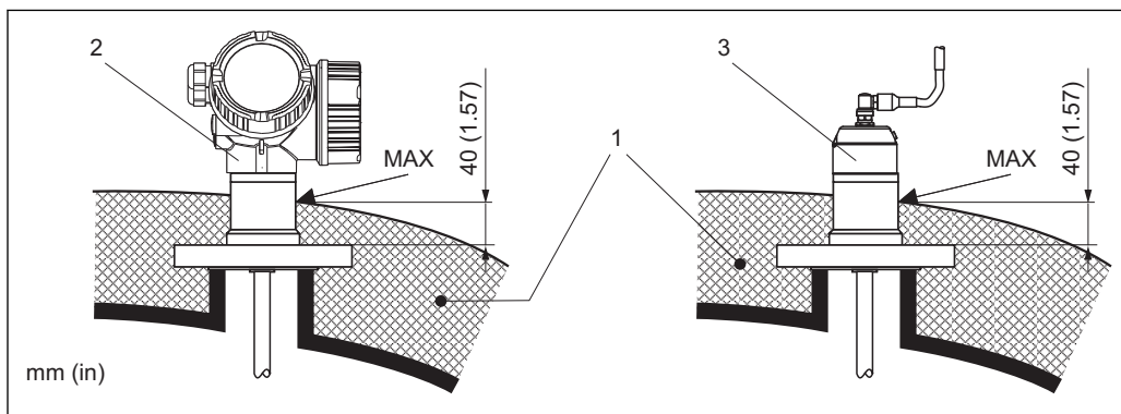
8 Фланцевое присоединение к процессу – FMP51
