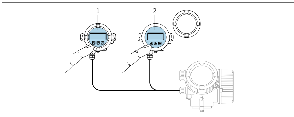
13 Варианты управления FHX50
