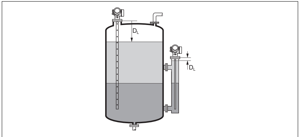
31 Расстояние для измерения уровня границы раздела фаз
