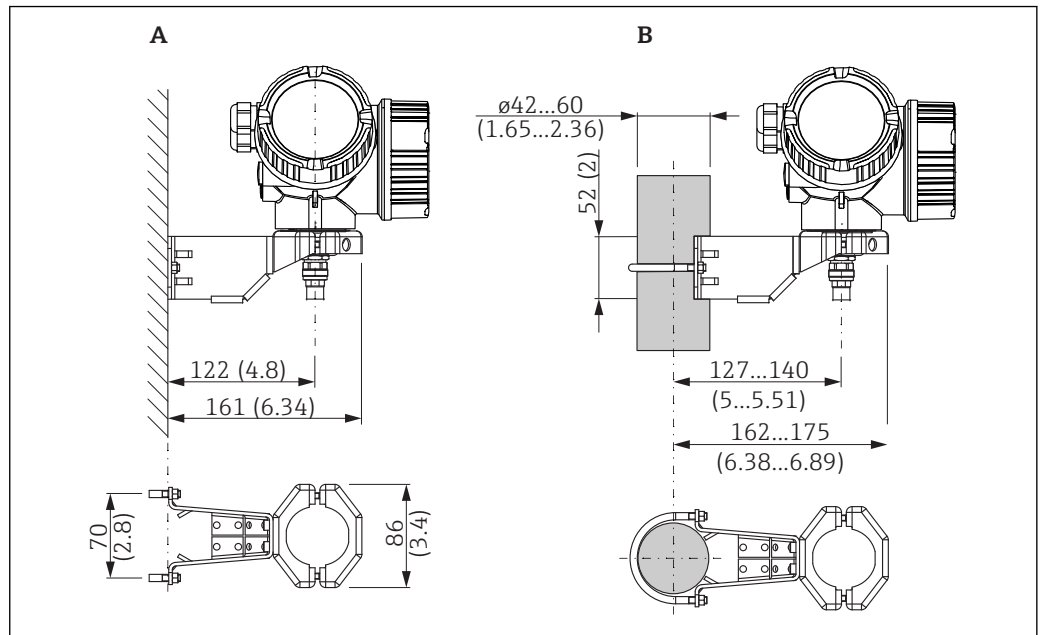
9 Монтаж корпуса электронной части с использованием кронштейна; размеры: мм (дюйм)
