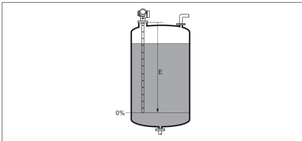
24 Калибровка пустой емкости (E) для измерения уровня жидких сред
