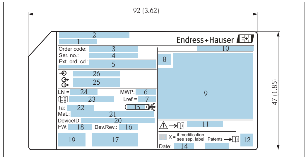
3 Заводская табличка Levelflex; размеры: мм (дюйм)
