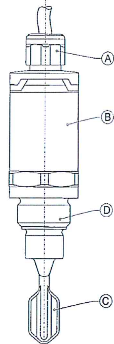
Liquiphant mit Kabelschwanz-Version
