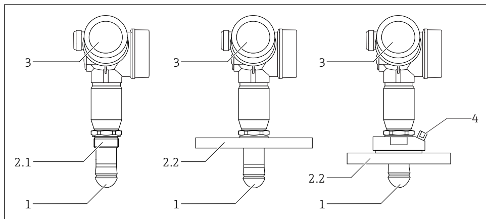
1 Konstrukce zařízení Micropilot FMR67
