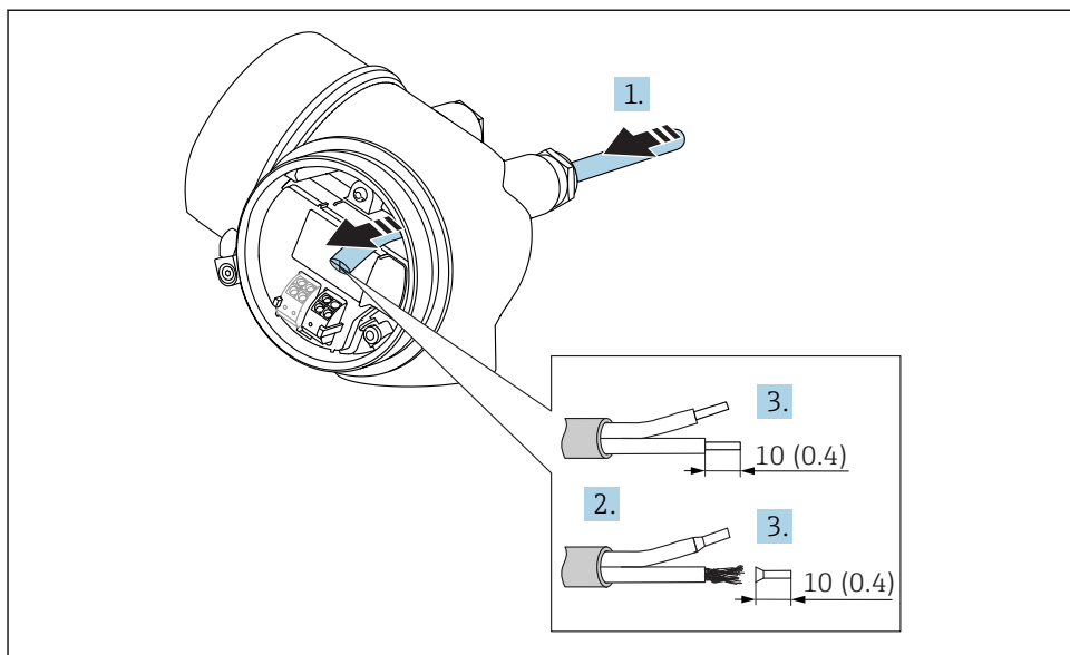
12 Rozměry: mm (in)
