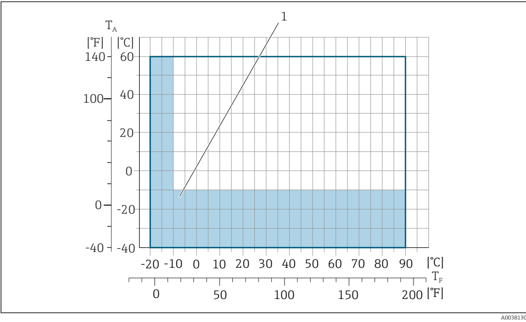
T_A Campo di temperatura ambiente T_F Temperatura del fluido 1 Area colorata: il campo di temperatura ambiente di -10 ... -40 °C (+14 ... -40 °F) e il campo di temperatura del fluido -10 ... -20 °C (+14 ... -4 °F) sono validi solo per flange in acciaio inox
