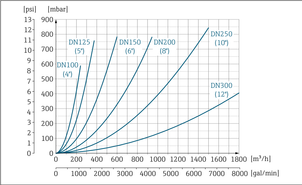
35 Perdita di carico DN 100 ... 300 (4 ... 12") per codice d'ordine per "Design", opzione C "Flangia fissa, senza tratti rettilinei in entrata/uscita"
