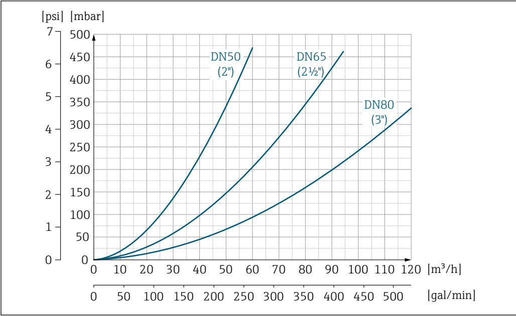
34 Perdita di carico DN 50 ... 80 (2 ... 3") per codice d'ordine per "Design", opzione C "Flangia fissa, senza tratti rettilinei in entrata/uscita"
