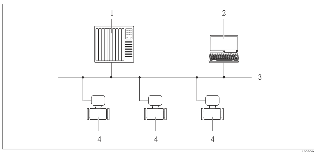
23 Opzioni per il funzionamento a distanza mediante rete PROFIBUS DP
