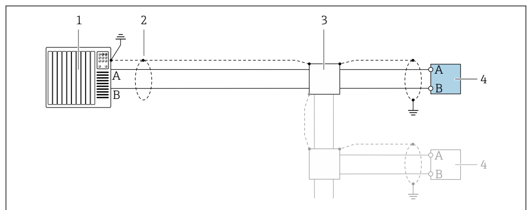
11 Esempio di connessione per PROFIBUS DP, area sicura e Zona 2/Div. 2
