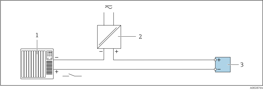
18 Esempio di connessione per ingresso di stato 1 Sistema di automazione con uscita di stato (ad es. PLC) 2 Alimentazione 3 Trasmettitore
