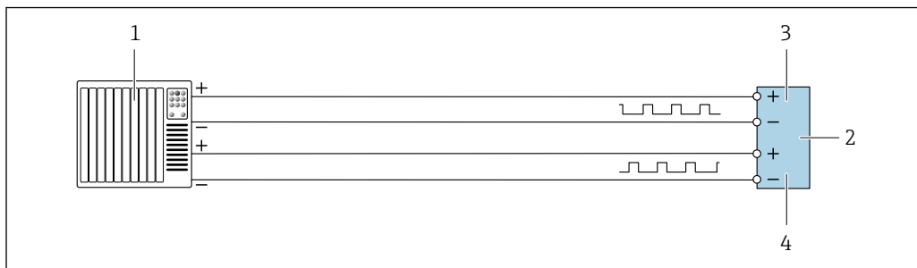
図 17 二重パルス出力（アクティブ）の接続例
