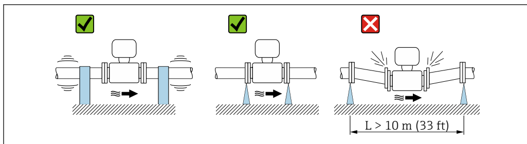
図 5 機器の振動を防止するための対策
