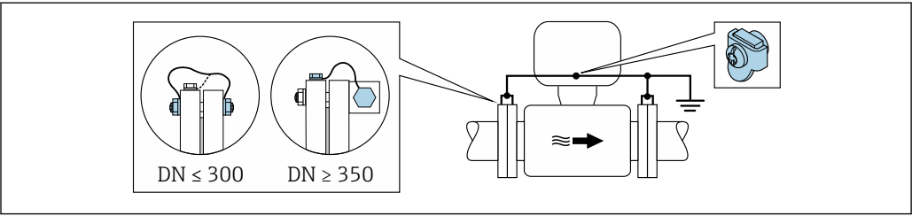
図 8 接地端子および配管フランジを介した電位平衡
