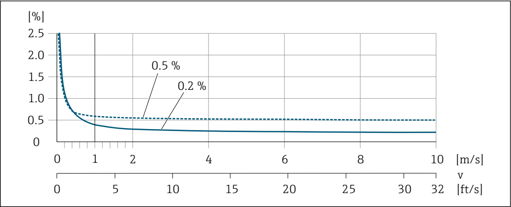
36 最大測定誤差 (%) o.r.
