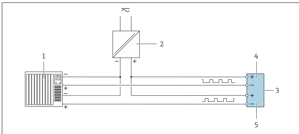
図 18 二重パルス出力（パッシブ）の接続例
