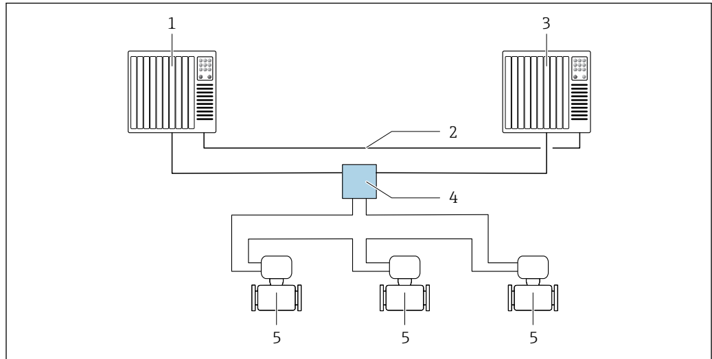
図 23 冗長システム (S2) のレイアウト例：リングトポロジー
