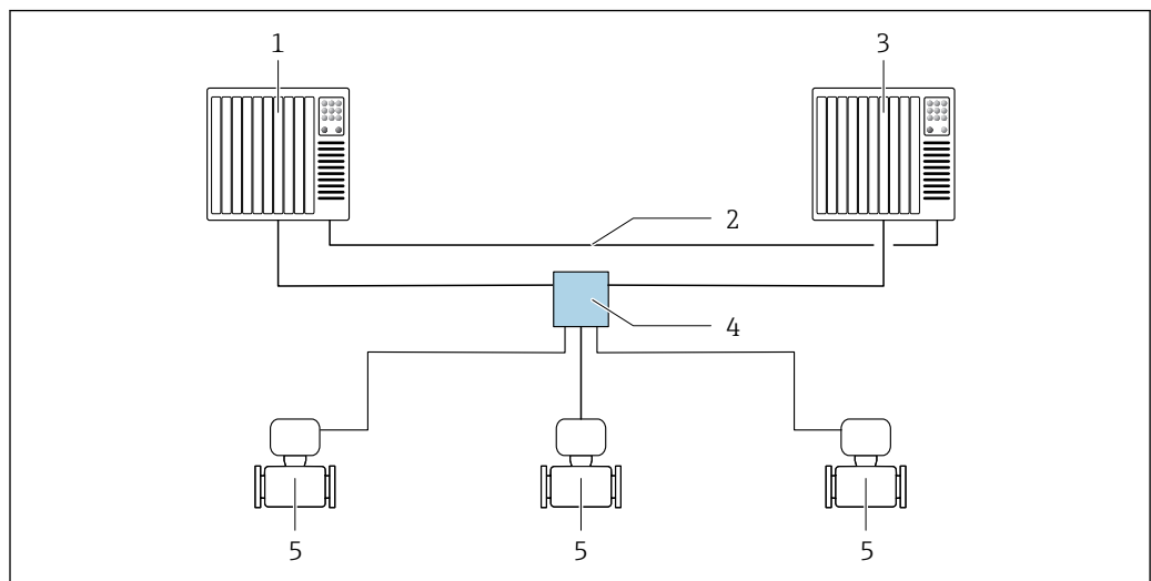
図 24 冗長システム (S2) のレイアウト例：スター型トポロジー
