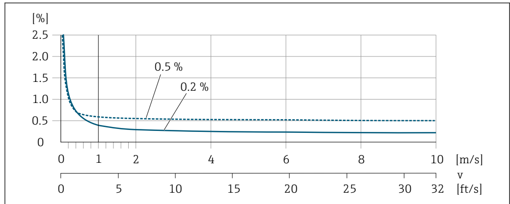
図 31 最大測定誤差 (%) o.r.
