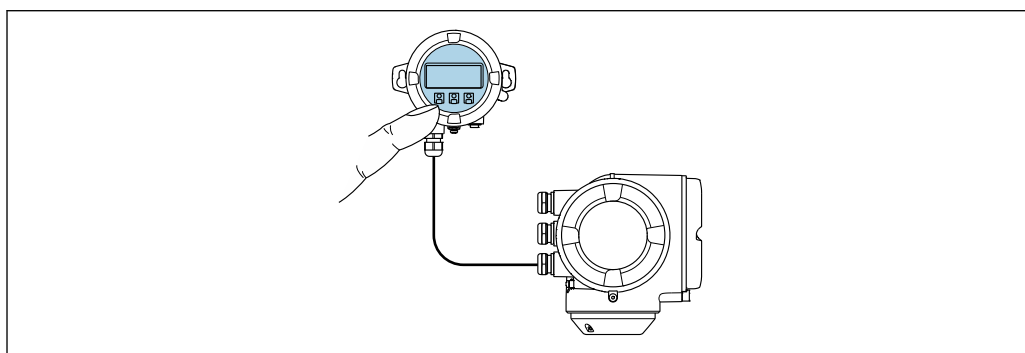
図 33 分離ディスプレイと操作モジュール DKX001 を介した操作
