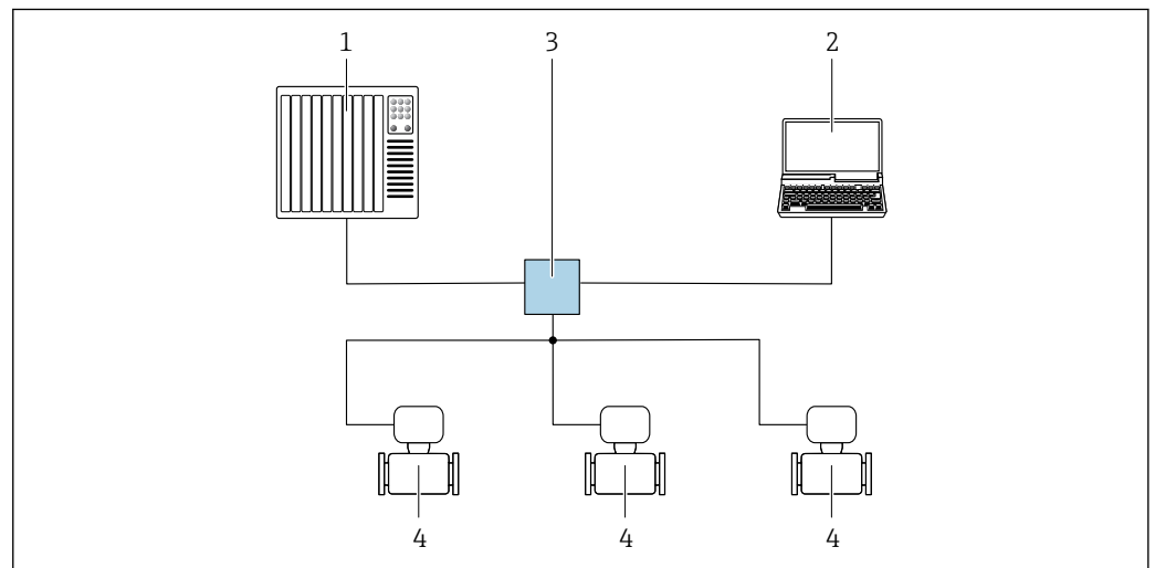
図 20 PROFINET ネットワーク経由のリモート操作オプション：スター型トポロジー
