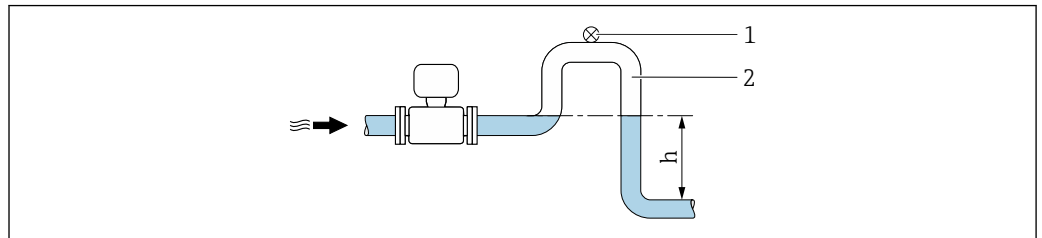
図 4 下向きの配管への設置
