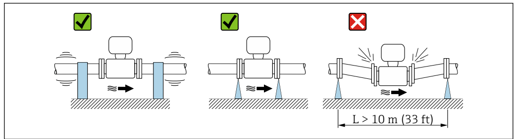
図 5 機器の振動を防止するための対策
