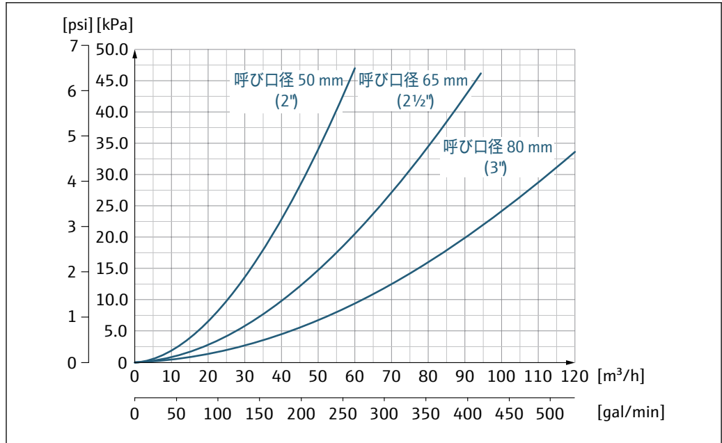
図 34 呼び口径 50～80 mm (2～3") の圧力損失：「設計」のオーダーコード、オプション C「固定フランジ、上流側/下流側直管長なし」の場合
